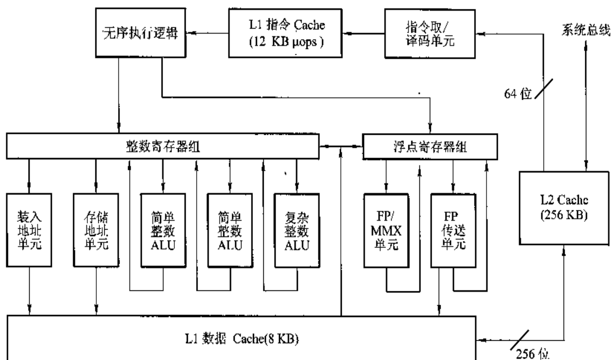
图 4.52 Pentium 4 处理器框图
