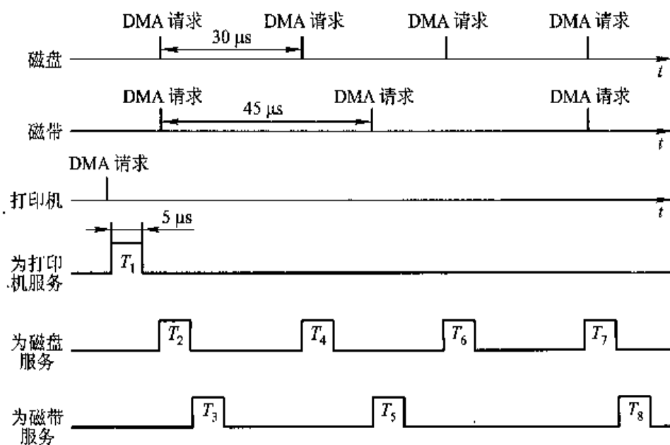
图 5.52 多路型 DMA 接口工作原理示意图
