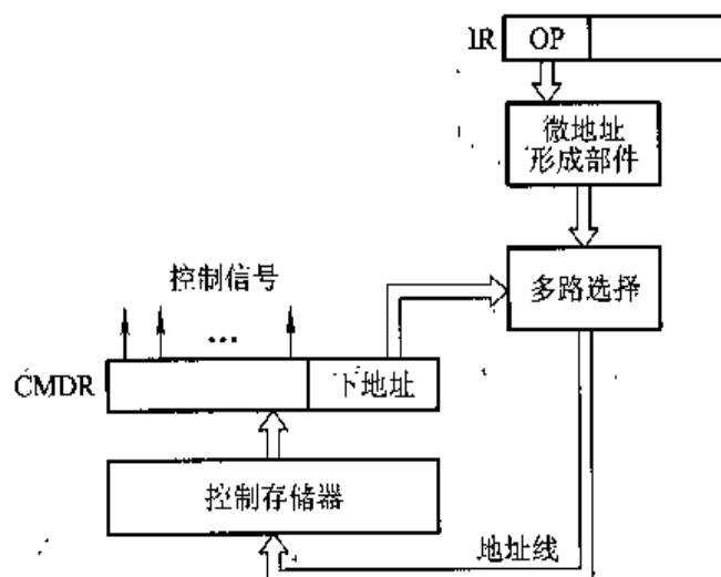
图 10.16 省去了 CMAR 的控制存储器
