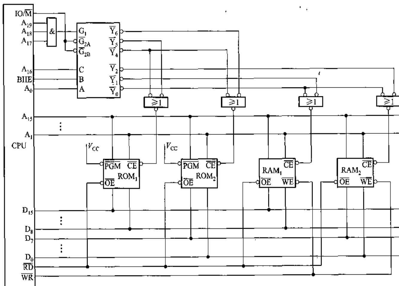
图 4.40 例 4.3 CPU 与存储芯片的连接图
