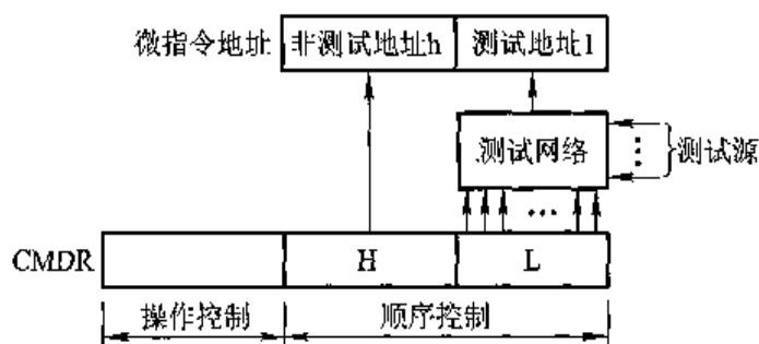
图 10.10 通过测试网络形成微指令地址
