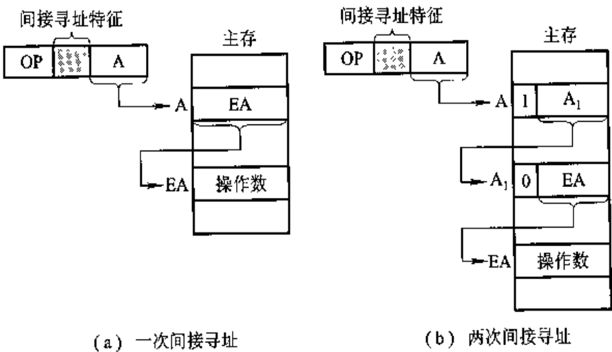
图 7.11 间接寻址示意图
