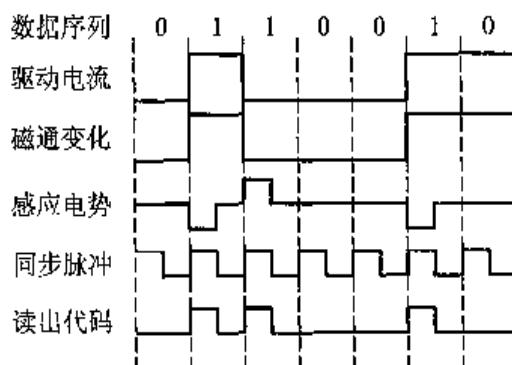
图 4.64 NRZI 的读出代码波形
