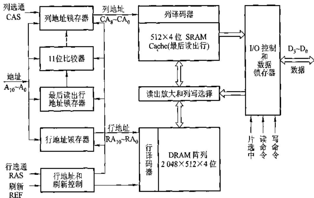
图 4.48 1\text{M} \times 4 位 CDRAM 芯片结构框图
