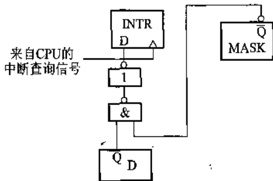
图 5.37 接口电路中 D、INTR、MASK 和中断查询信号的关系
