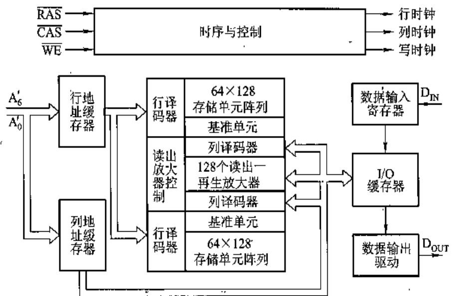
图 4.20 4116 动态 RAM (16 K × 1 位) 芯片的结构
