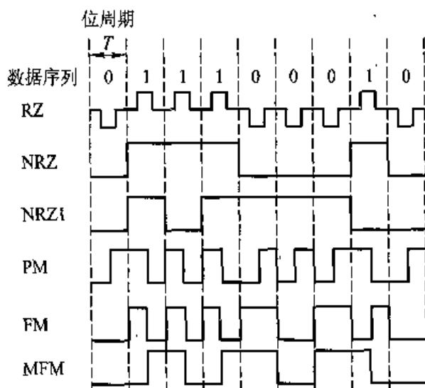
图 4.63 六种磁记录方式的写入电流波形
