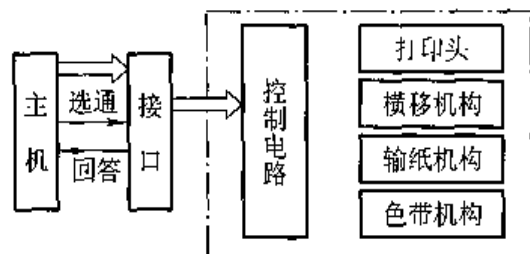
(a) 针式打印机结构框图
