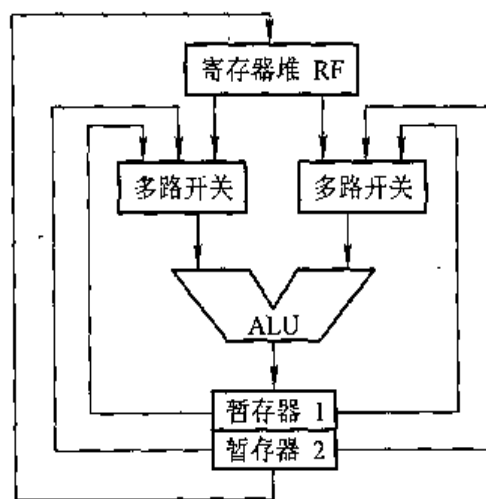
图 8.16 带有旁路技术的 ALU 部件
