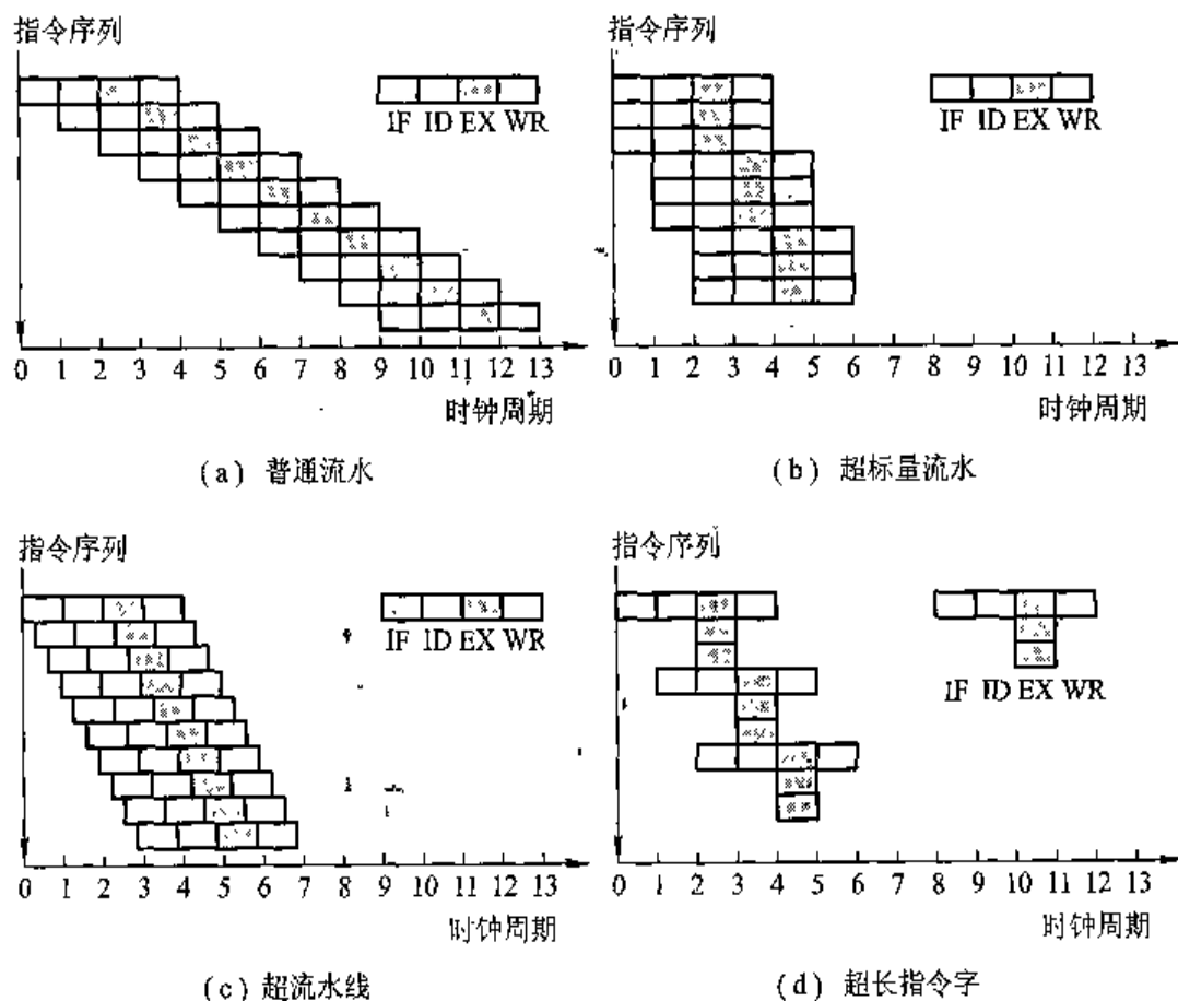
图 8.20 四种流水技术的比较
