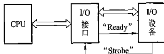
图 5.6 异步并行“应答”联络方式
