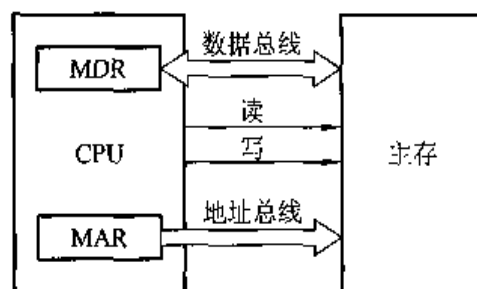
图 4.5 主存和 CPU 的联系
