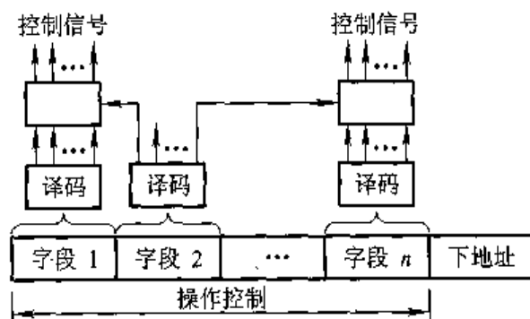
图 10.9 字段间接编码方式
