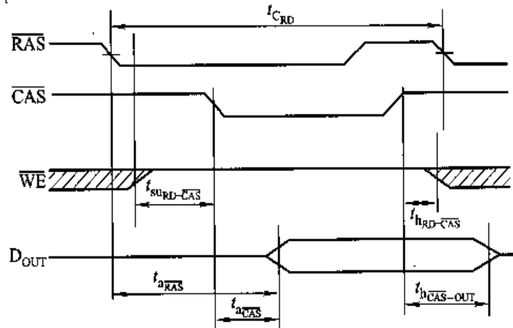
图 4.22 动态 RAM 读工作方式时序图
