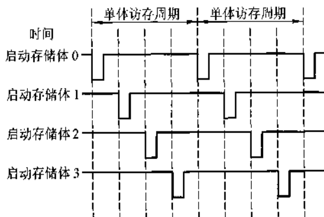
图 4.44 4 个存储体交叉访问的时间关系
