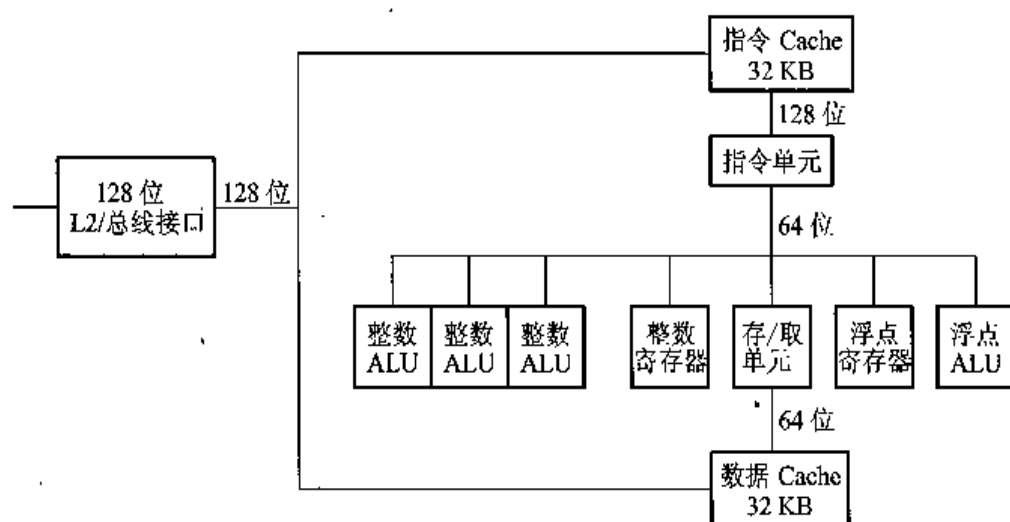
图 4.53 PowerPC 620 处理器框图
