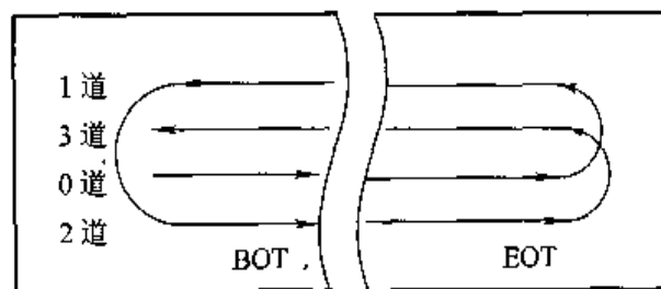
图 4.77 4 道 1/4 英寸磁带蛇形串行记录方式
