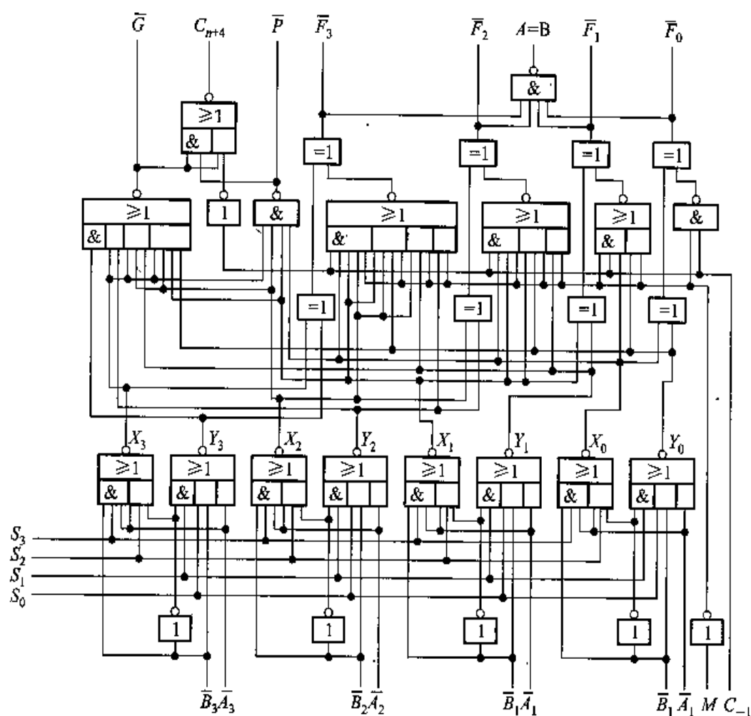
图 6.30 负逻辑操作数表示的 74181 ALU 电路
