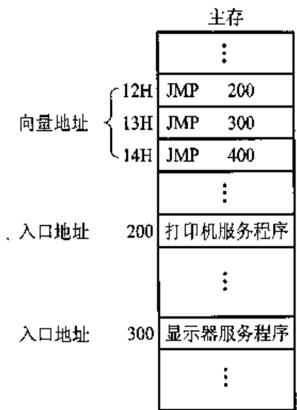
图 5.40 通过向量地址寻找入口地址
