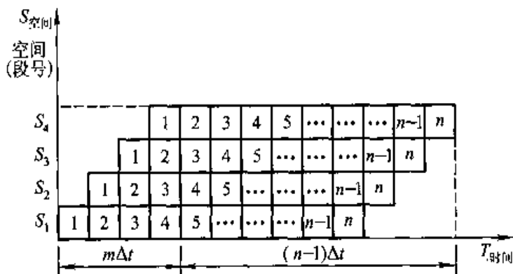
图 8.18 各段时间相等的流水线时空图
