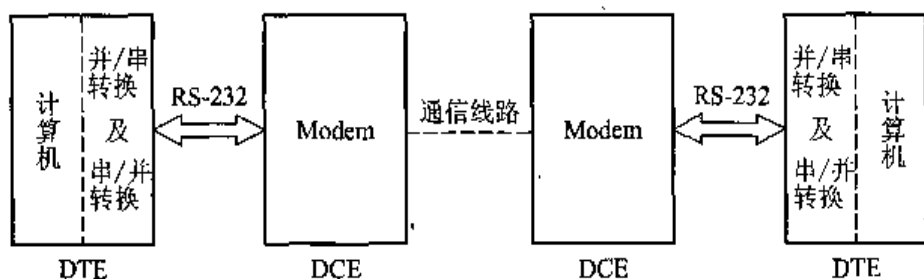
图 3.5 串行通信系统
