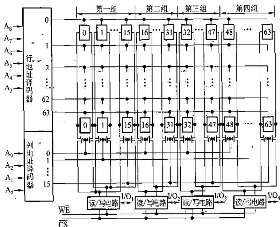
图 4.14 2114 RAM 矩阵结构示意图
