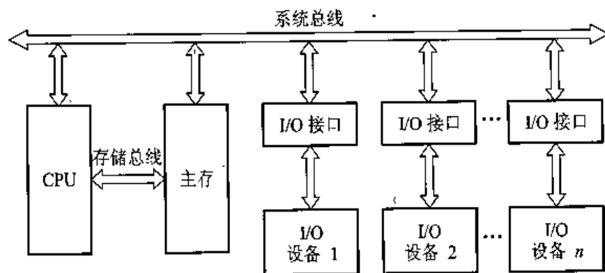
图 3.3 以存储器为中心的双总线结构框图
