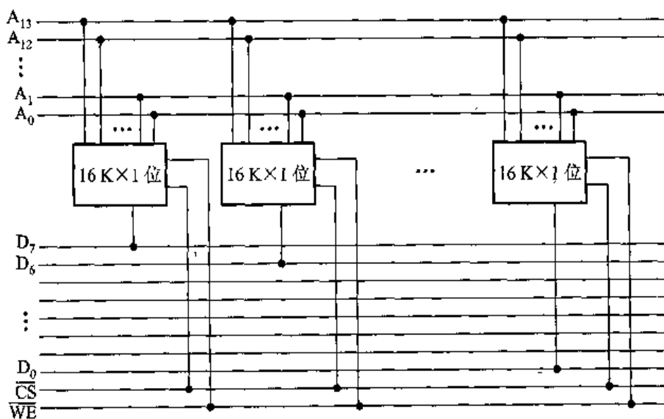
图 4.33 由 8 片 16\text{ K} \times 1 位的芯片组成 16\text{ K} \times 8 位的存储器
