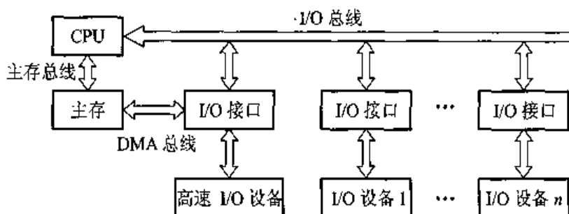
图 3.8 三总线结构
