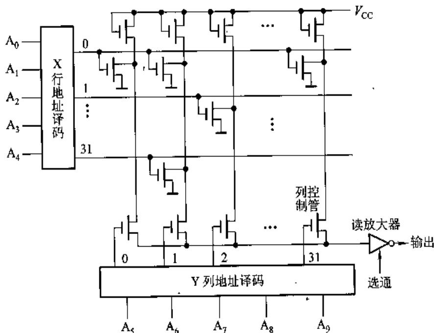
图 4.27 1K \times 1 位的 MOS 管掩模 ROM
