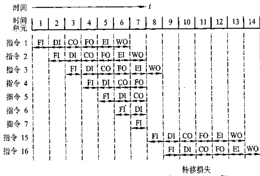
图 8.17 条件转移对指令流水操作的影响
