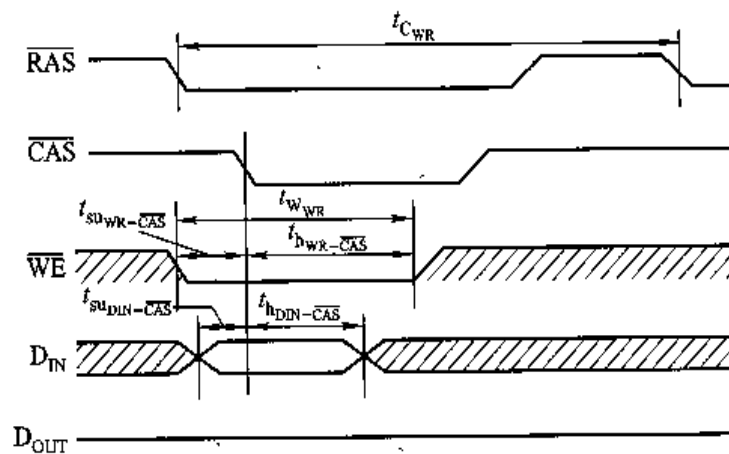
图 4.23 动态 RAM 写工作方式时序图
