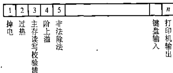
图 8.24 中断请求标记寄存器
