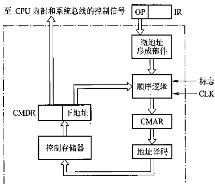
图 10.5 微程序控制单元的基本组成
