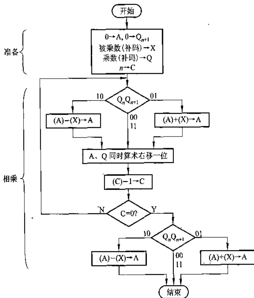
图 6.10 补码一位乘比较法控制流程图
