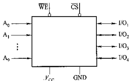
图 4.12 Intel 2114 外特性示意图
