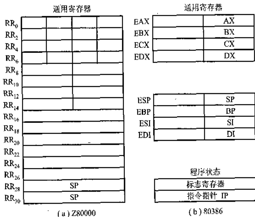
图 8.4 两种 32 位微处理器寄存器组织
