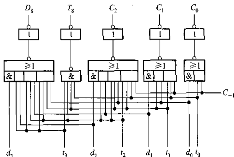
图 6.25 双重分组跳跃进位链的小组进位线路
