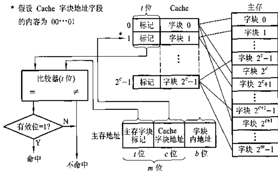
图 4.54 直接映射
