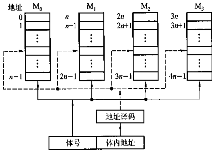
图 4.42 高位交叉编址的多体存储器
