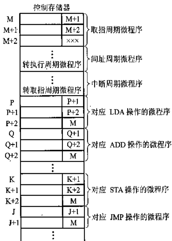
图 10.4 不同机器指令所对应的微程序
