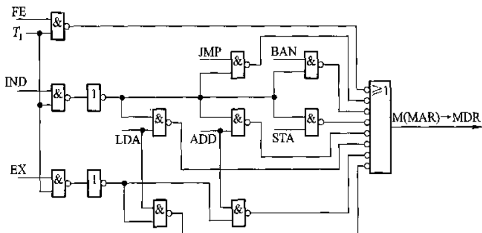
图 10.3 产生 M(\text{MAR}) \rightarrow \text{MDR} 命令的逻辑图
