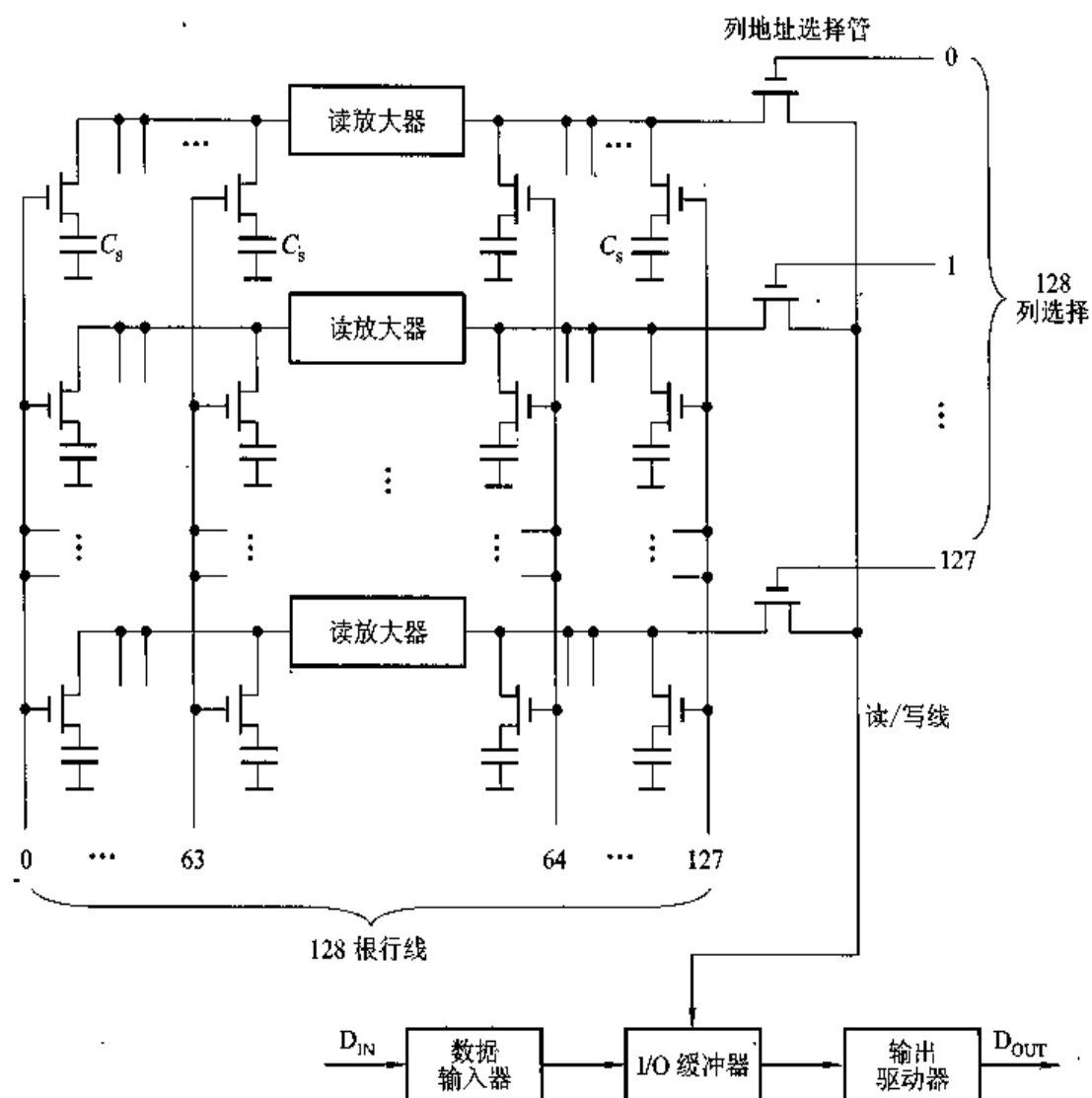
图 4.21 16 K × 1 位 4116 动态 RAM 存储矩阵示意图
