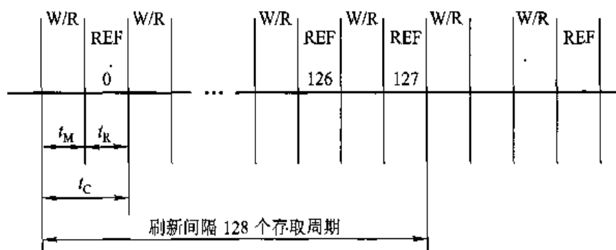
图 4.25 分散刷新时间分配示意图
