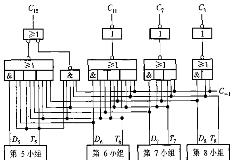
图 6.24 双重分组跳跃进位链的大组进位线路
