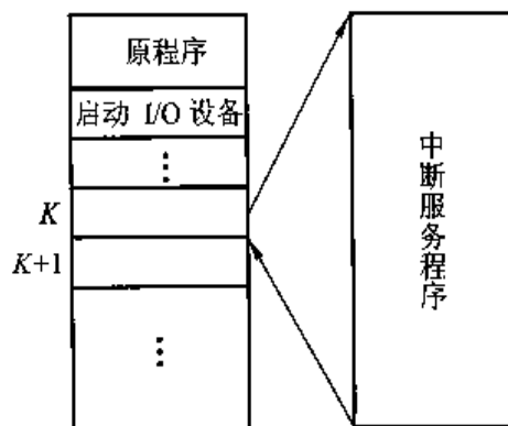
图 5.10 程序中断方式示意图
