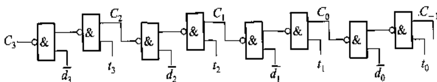
图 6.20 四位串行进位链
