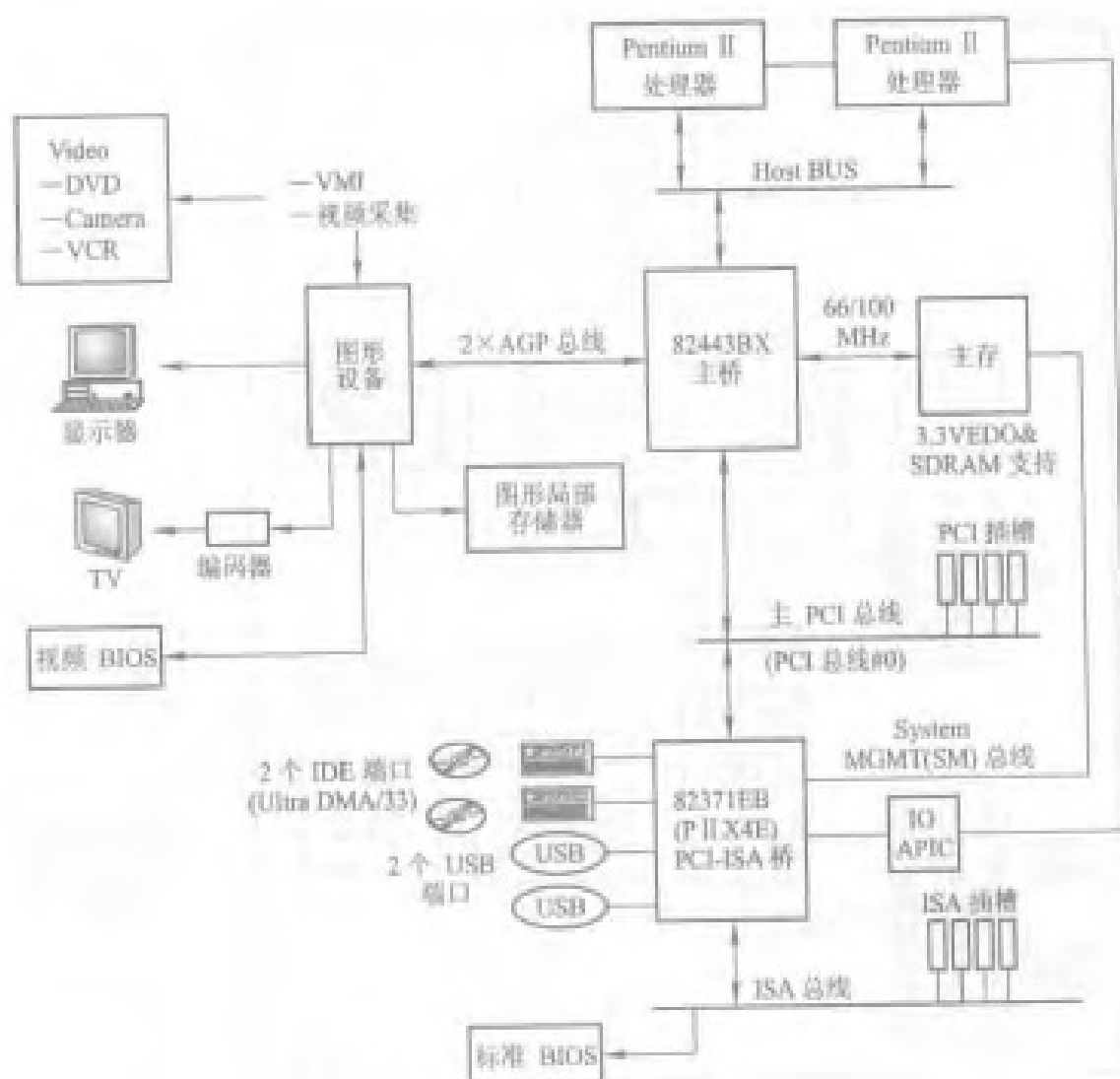
图 10.20 440 BX 主板结构示意图
