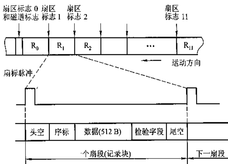
图 4.71 ISOT 型磁盘的磁道记录格式
