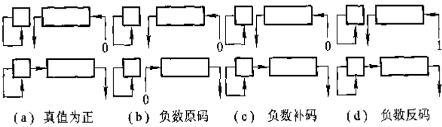
图 6.3 实现算术左移和右移操作的硬件示意图
