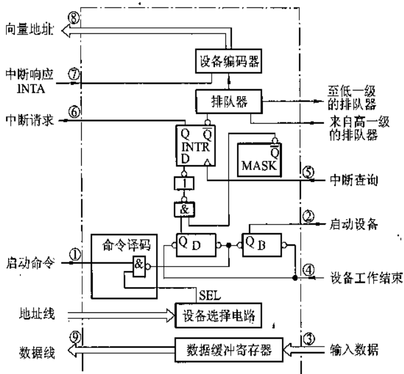
图 5.41 程序中断方式接口电路的基本组成
