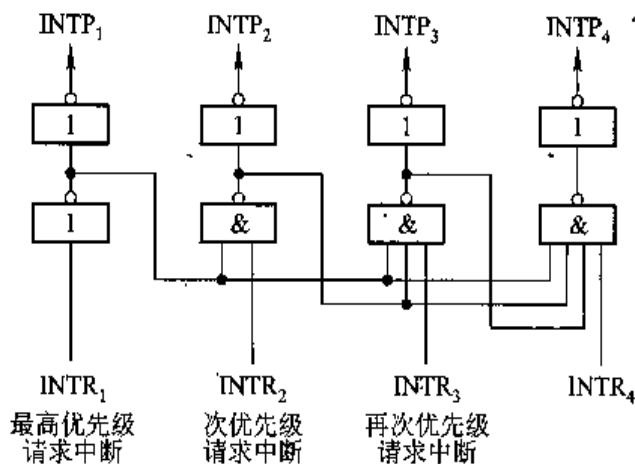
图 8.25 集中在 CPU 内的排队器
