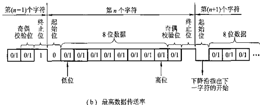
图 3.19 两种传输率的异步串行传送字符格式
