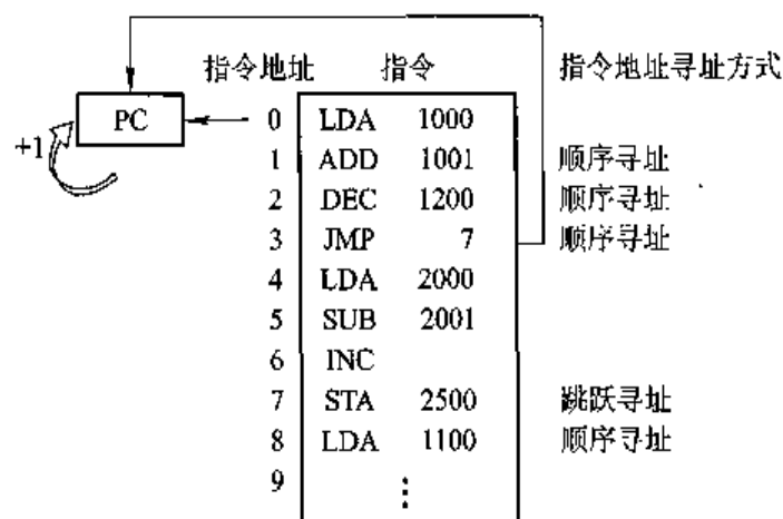
图 7.6 指令的寻址方式示意图
