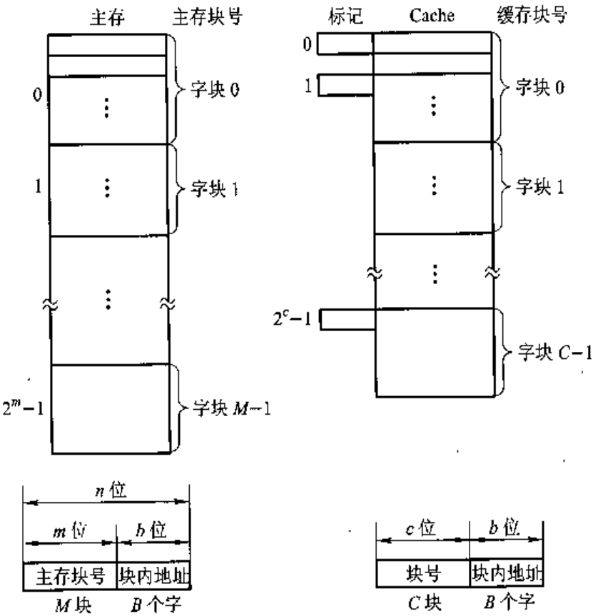
图 4.49 Cache - 主存存储空间的基本结构
