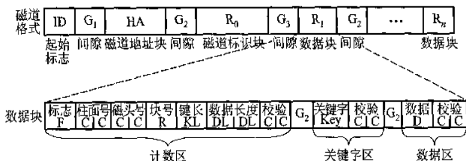
图 4.73 IBM 2311 盘不定长度磁道记录格式的示意图
