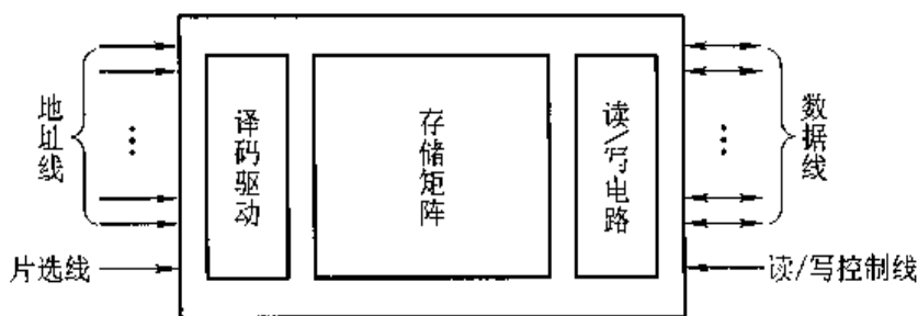
图 4.7 存储芯片的基本结构
