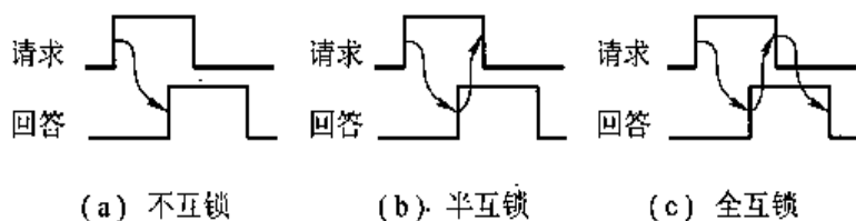
图 3.18 异步通信中请求与回答的互锁
