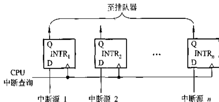
图 8.29 CPU 在统一时间发中断查询信号
