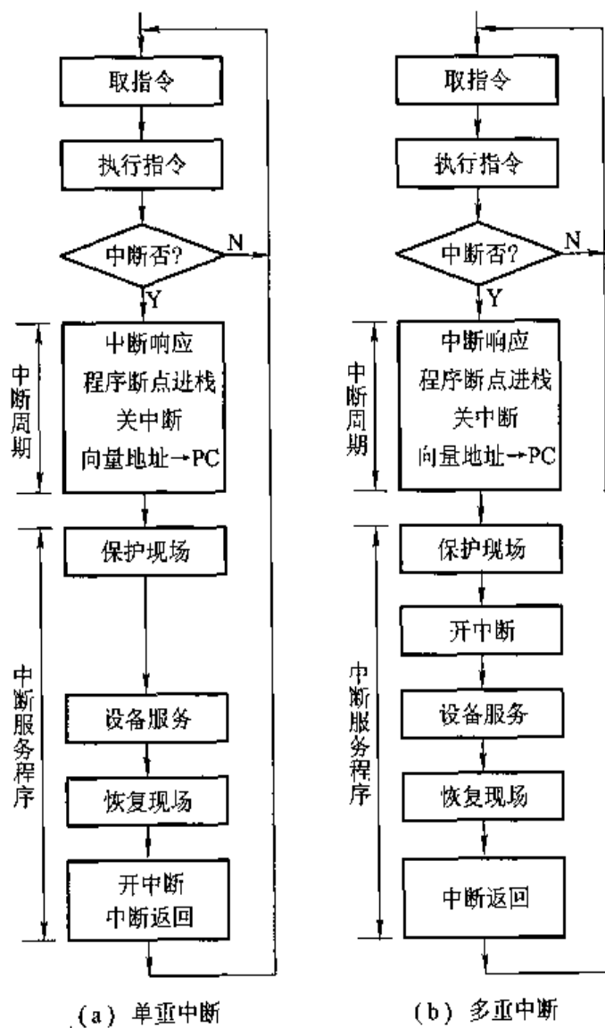
图 5.43 单重中断和多重中断服务程序流程
