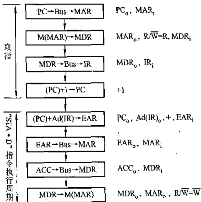
图 9.7 “STA * D”指令周期的信息流程及相应的控制信号
