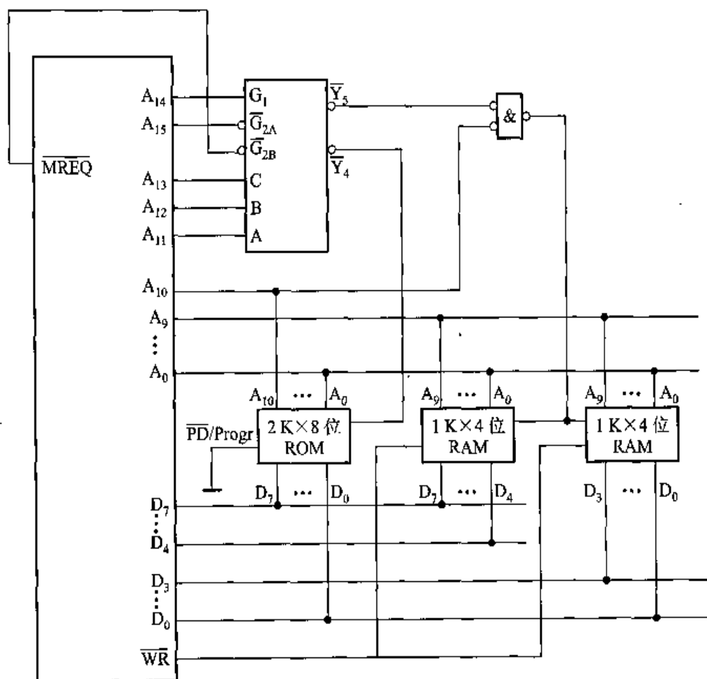
图 4.37 例 4.1 CPU 与存储芯片的连接图
