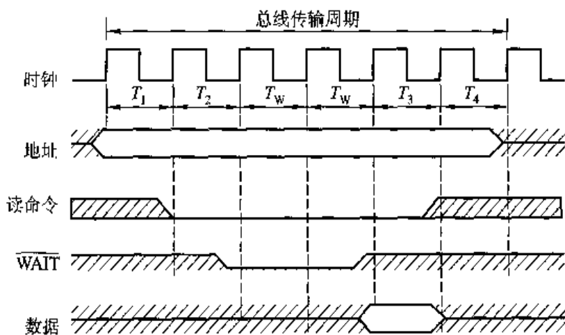
图 3.22 半同步通信数据输入过程
