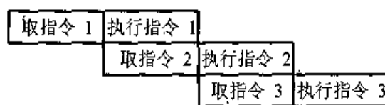
图 8.14 指令的二级流水
