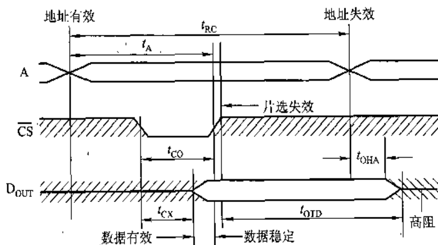
图 4.15 2114 RAM 的读周期时序
