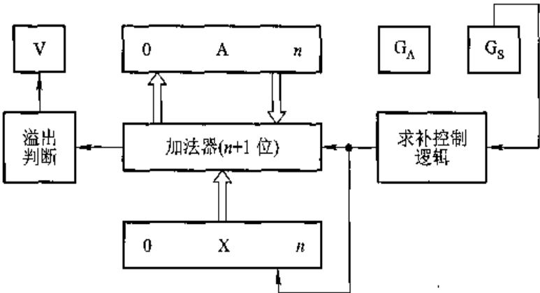
图 6.5 补码定点加减法硬件配置
