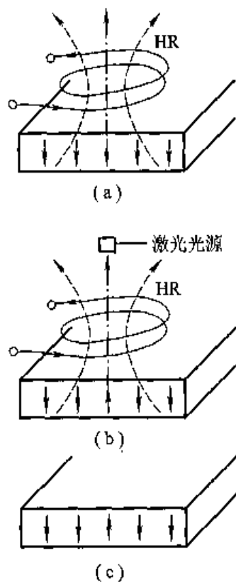
图 4.79 磁光记录原理
