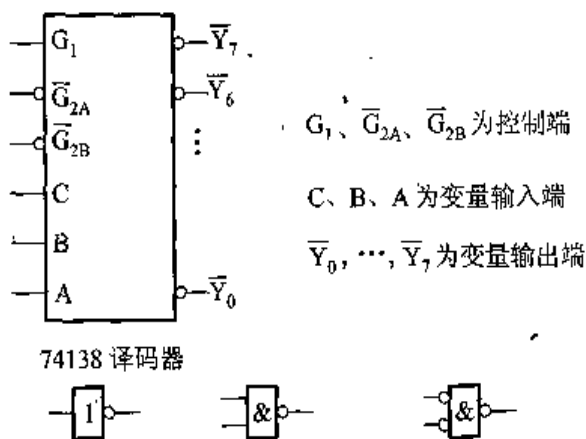
图 4.36 译码器和门电路
