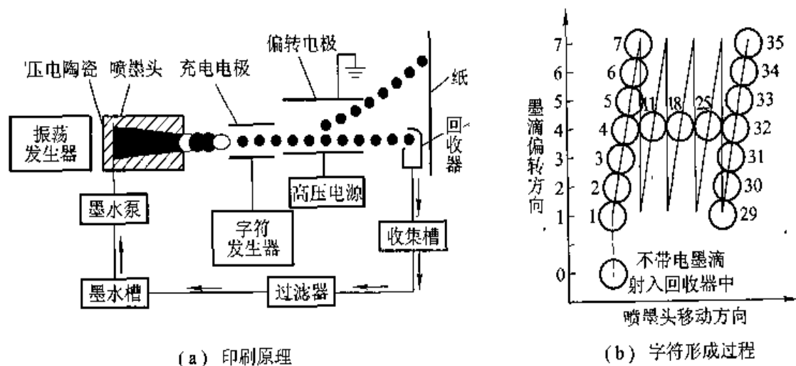
图 5.25 电荷控制式喷墨打印机原理框图
