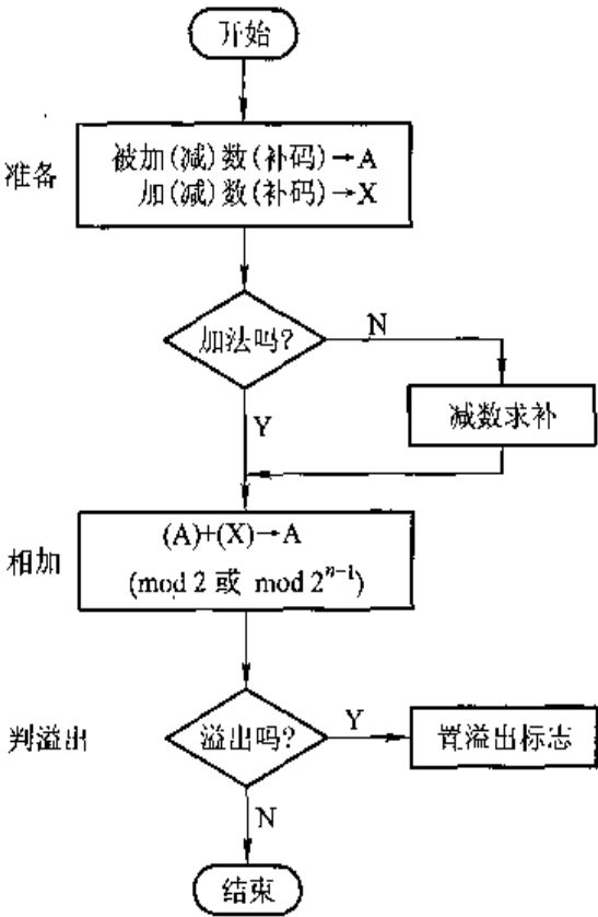
图 6.6 补码加减运算控制流程
