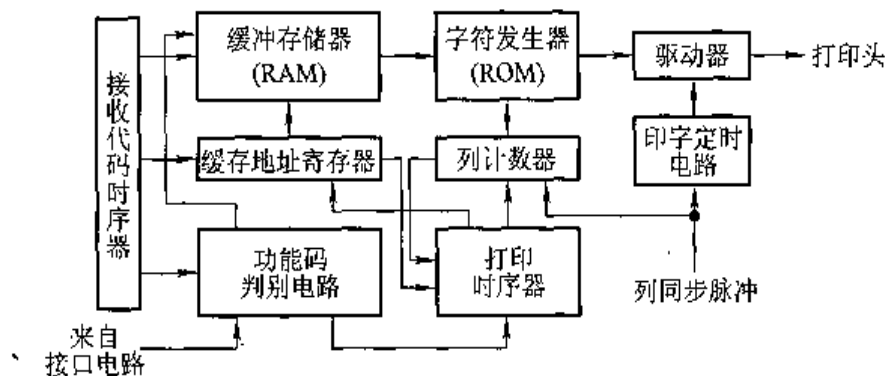
(b) 针式打印机控制电路框图
