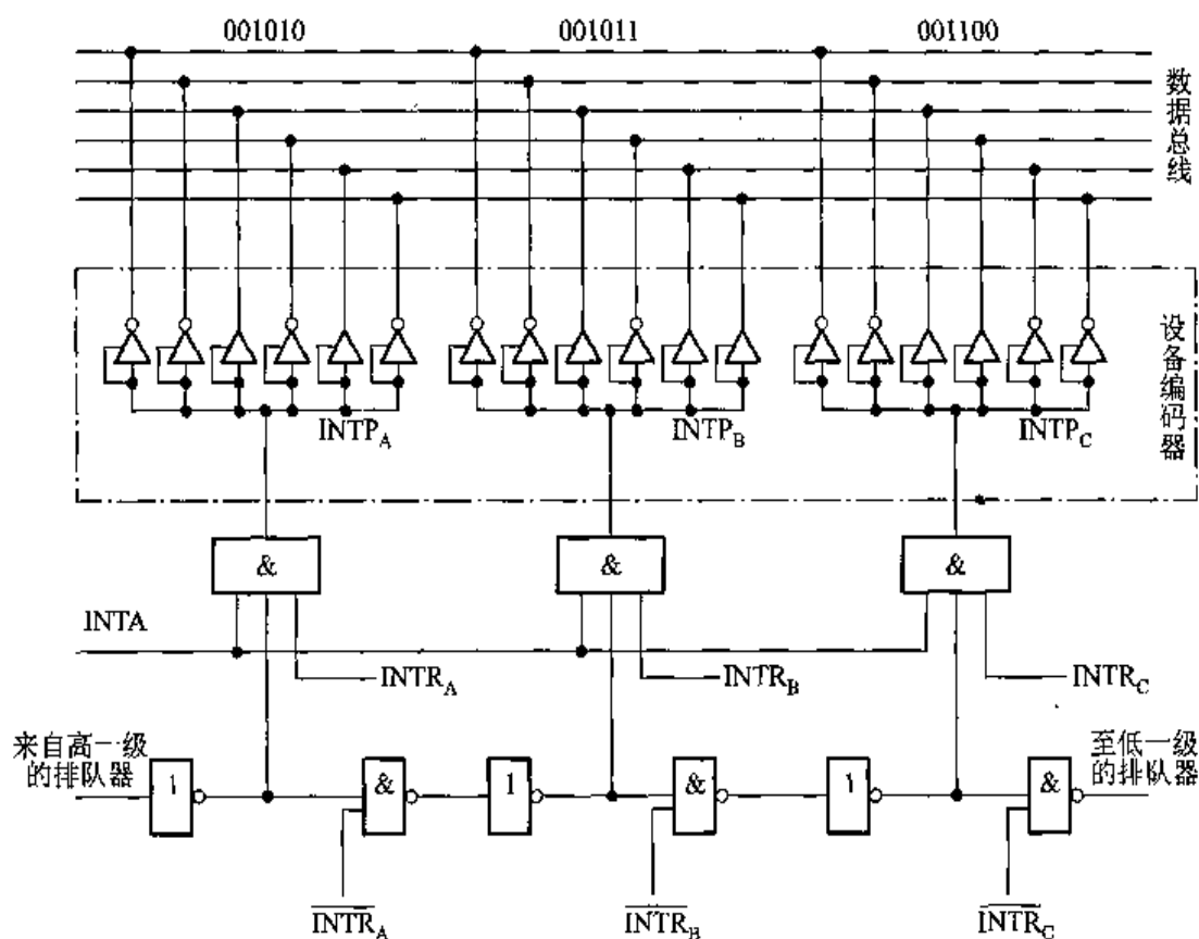
图 5.42 例 5.2 电路图
