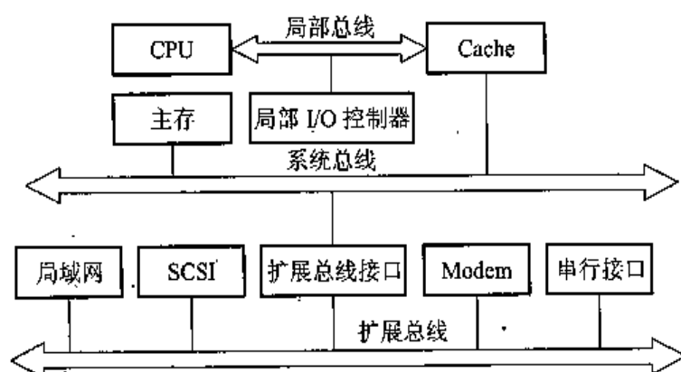
图 3.9 三总线结构的又一形式
