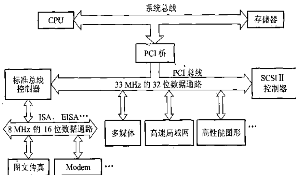
图 3.13 PCI 总线结构
