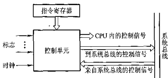
图 9.2 控制单元外特性
