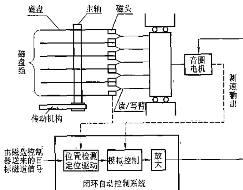
图 4.67 磁盘驱动器结构及定位驱动系统的示意图
