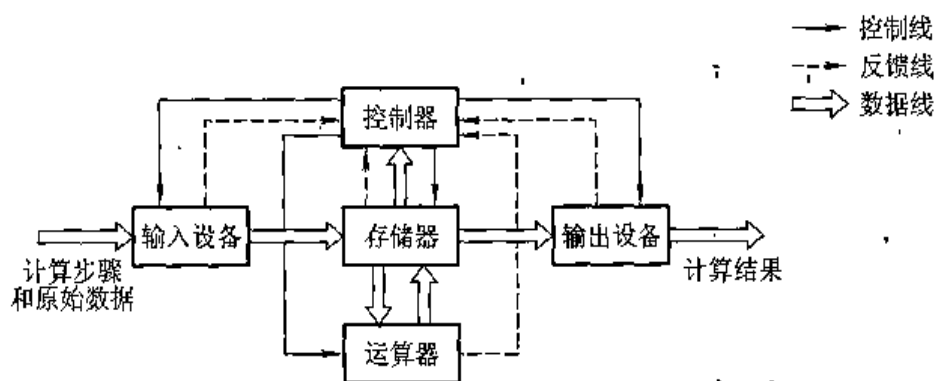
图 1.8 以存储器为中心的计算机结构框图
