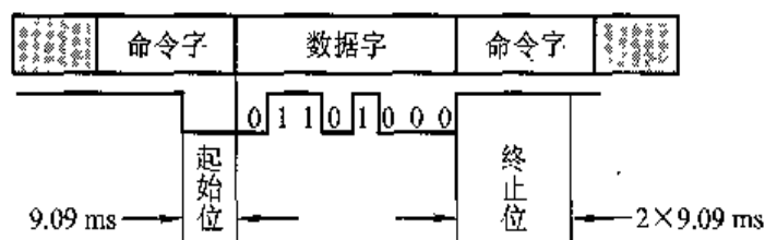
图 5.7 异步串行联络方式
