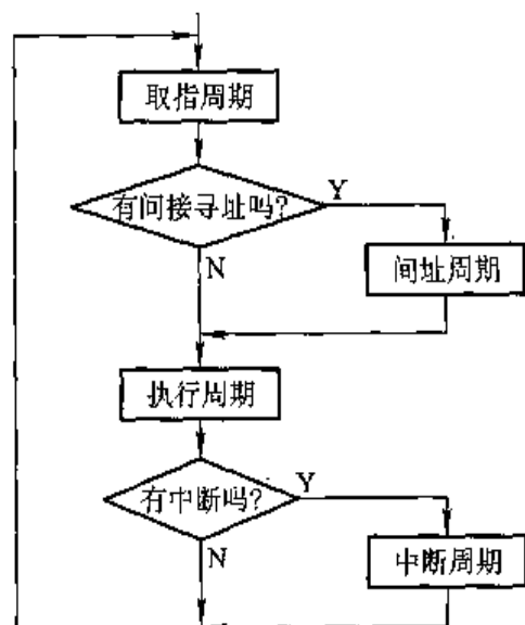
图 8.8 指令周期流程
