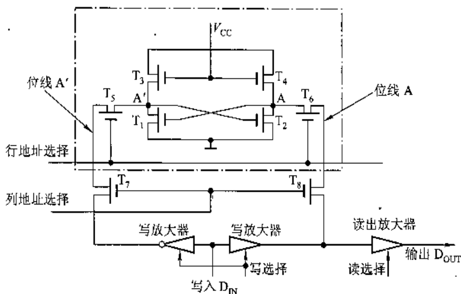
图 4.11 静态 RAM 的基本单元电路
