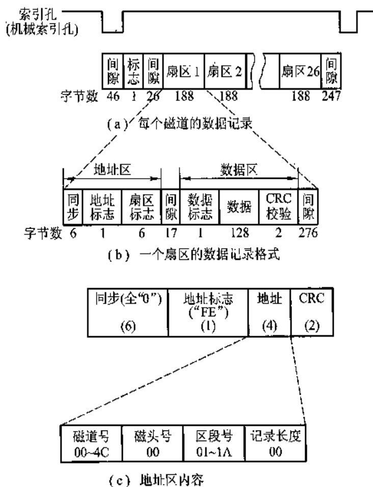
图 4.75 IBM 3740 软分段格式
