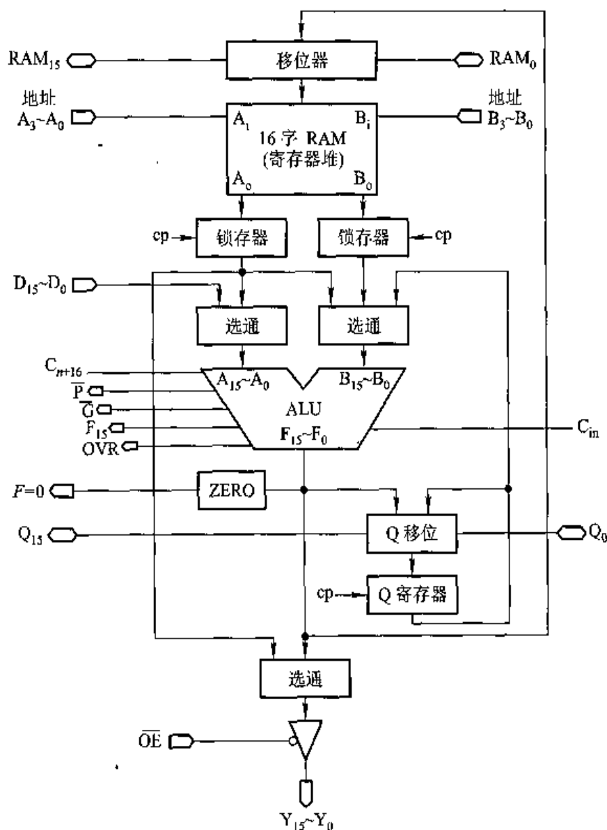
图 6.18 29C101 框图
