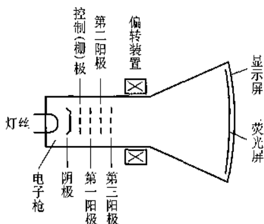
图 5.17 CRT 结构示意图
