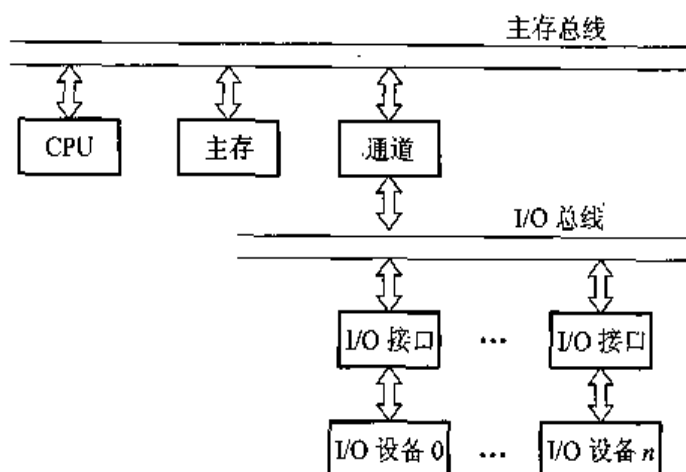
图 3.7 双总线结构
