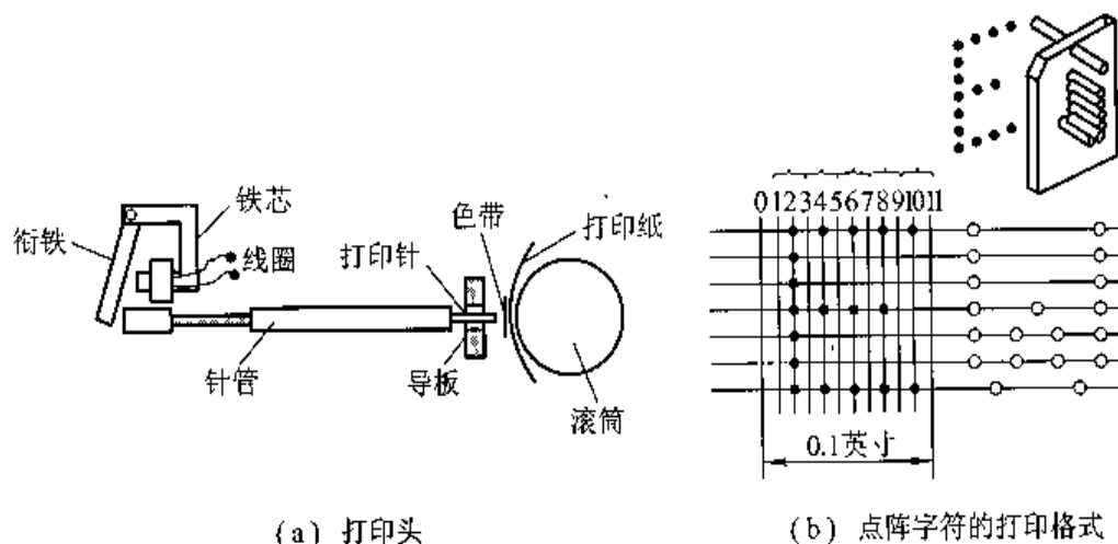
图 5.22 针式打印头和打印格式的示意图
