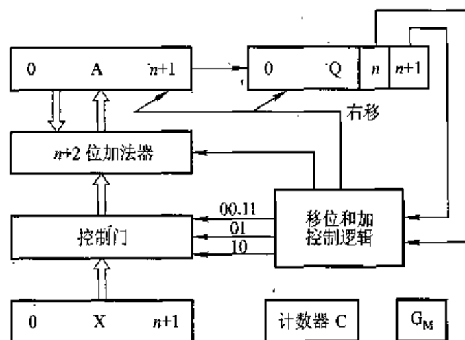
图 6.9 补码比较法运算基本硬件配置
