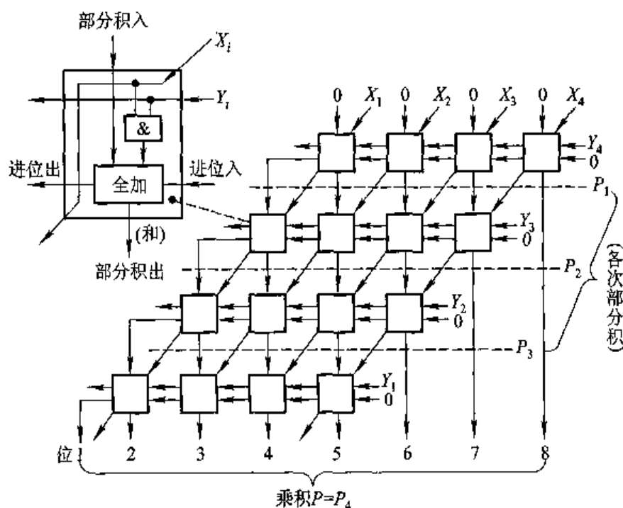
图 6.28 绝对值相乘的阵列乘法器
