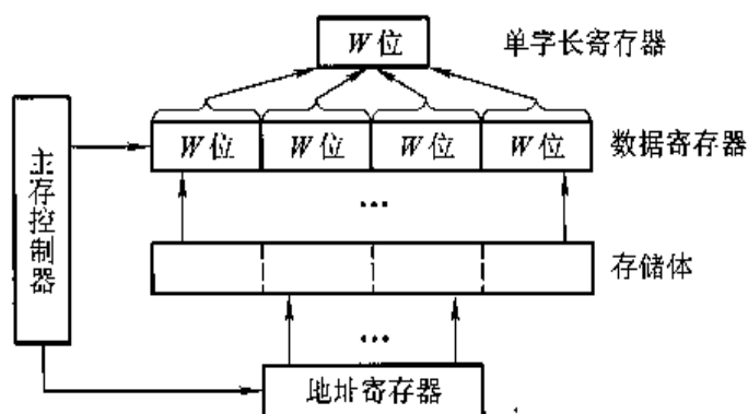
图 4.41 单体四字结构存储器
