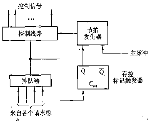
图 4.46 存控基本结构框图
