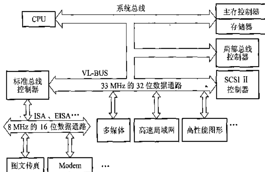
图 3.12 VL-BUS 局部总线结构
