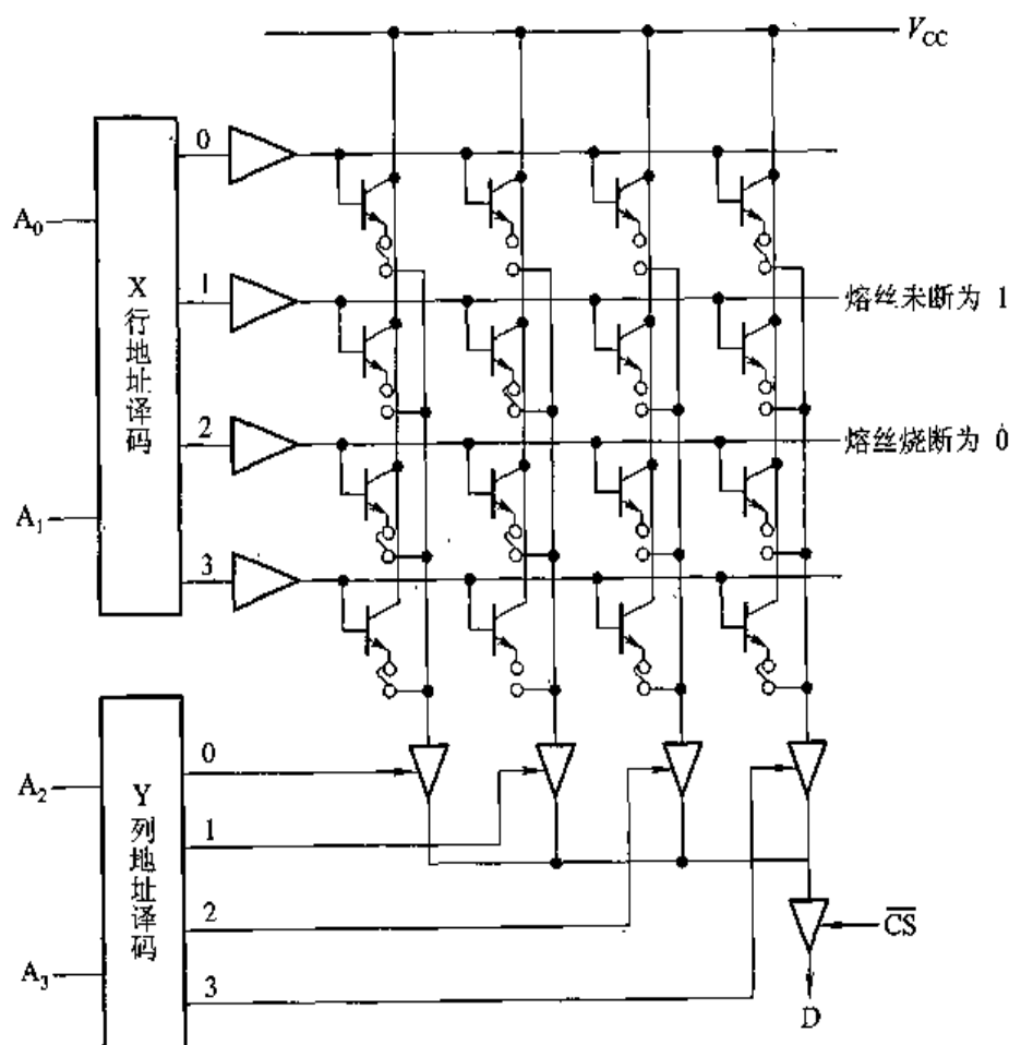
图 4.29 16 \times 1 位双极型镍铬熔丝式 PROM
