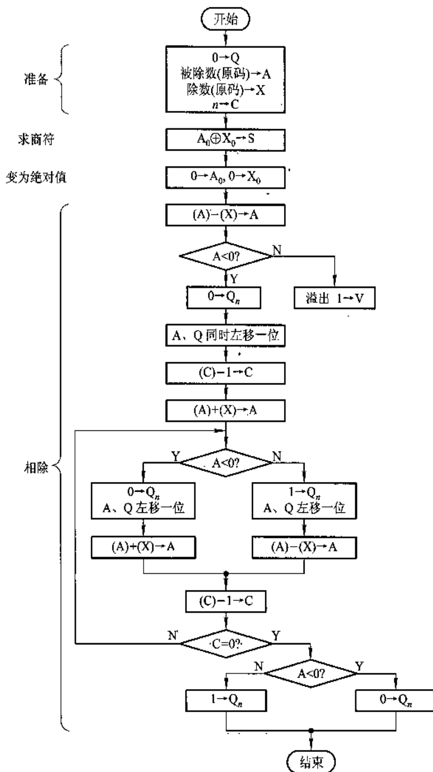
图 6.12 原码加减交替法控制流程图
