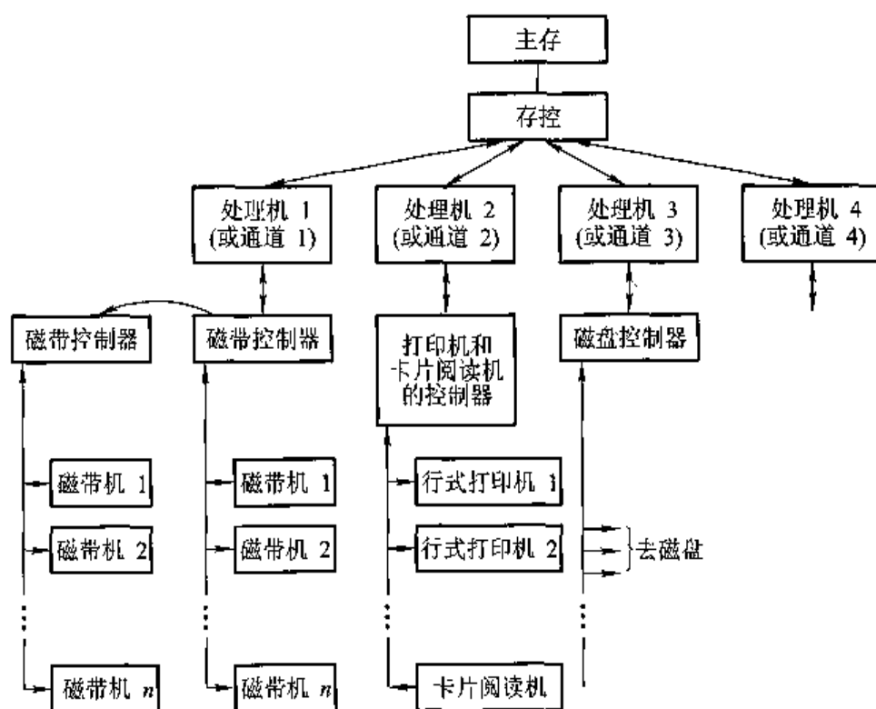
图 5.5 具有通道的 I/O 系统
