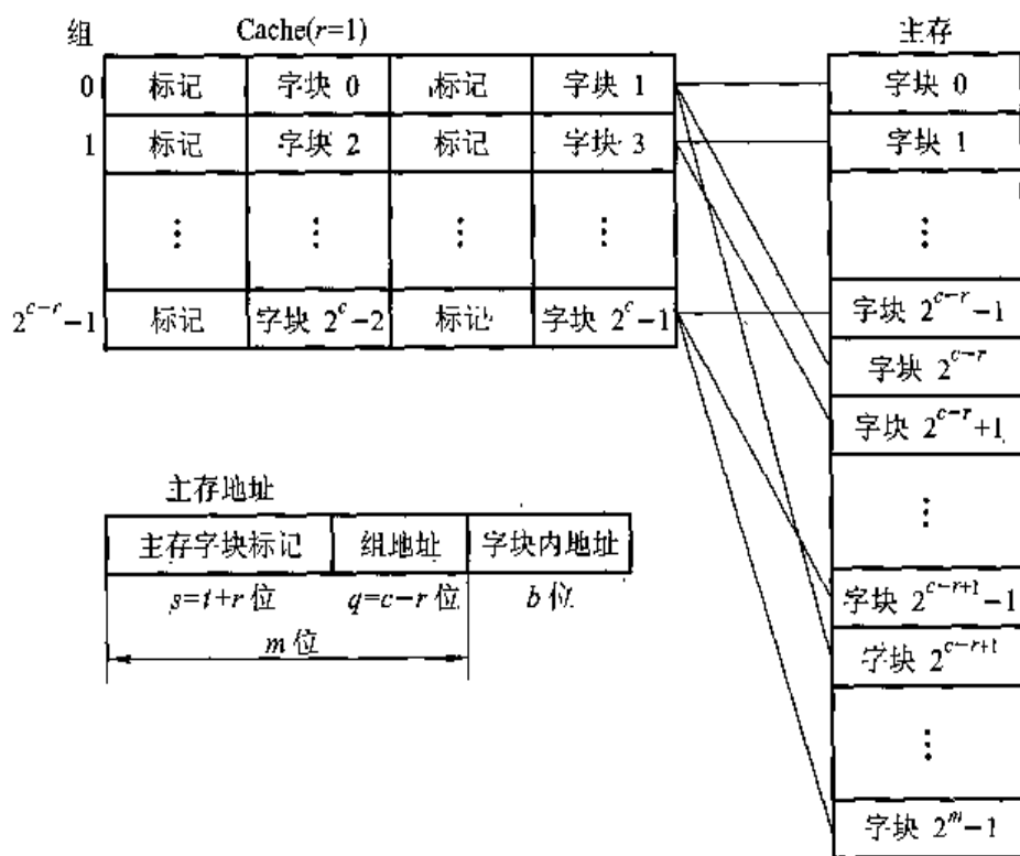
图 4.56 组相联映射
