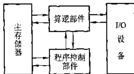
图 2.1 IAS 计算机结构
