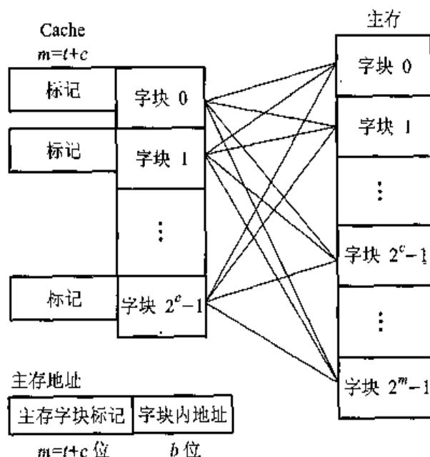
图 4.55 全相联映射
