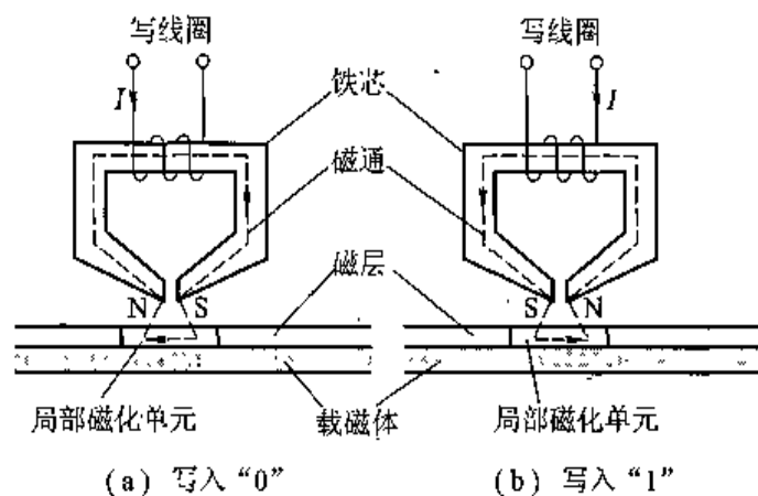
图 4.61 磁表面存储器写入原理
