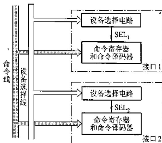
图 5.30 命令寄存器和命令译码器
