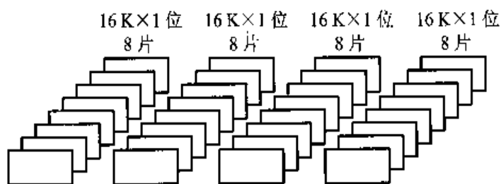
图 4.8 64 \text{ K} \times 8 位的存储器
