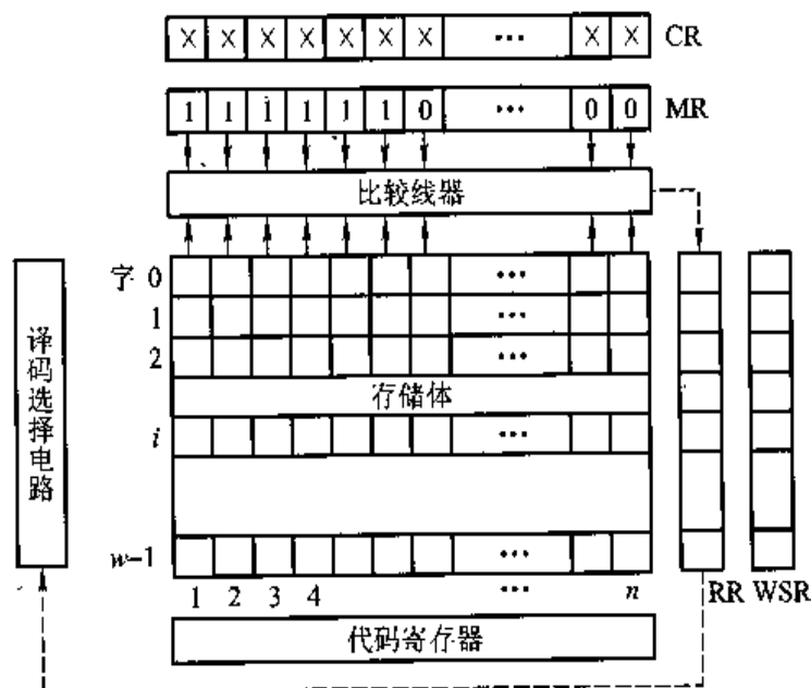
图 4.81 相联存储器基本组成框图
