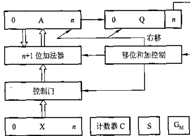
图 6.7 原码一位乘运算基本配置
