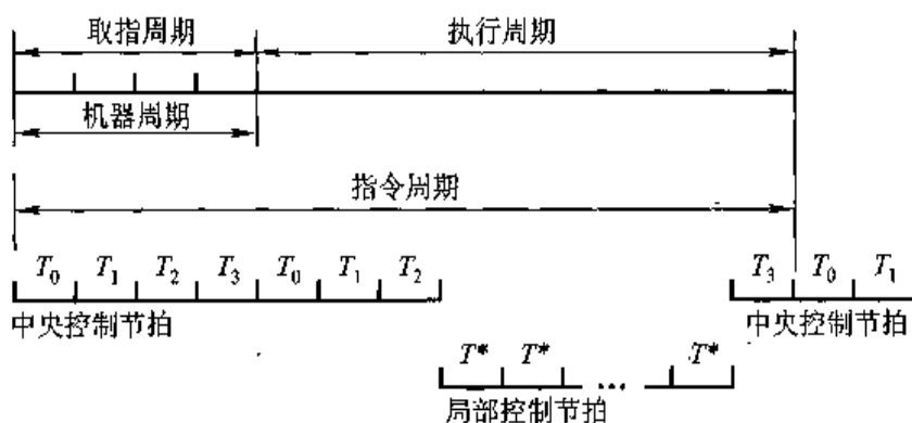
图 9.11 中央控制和局部控制的时序关系
