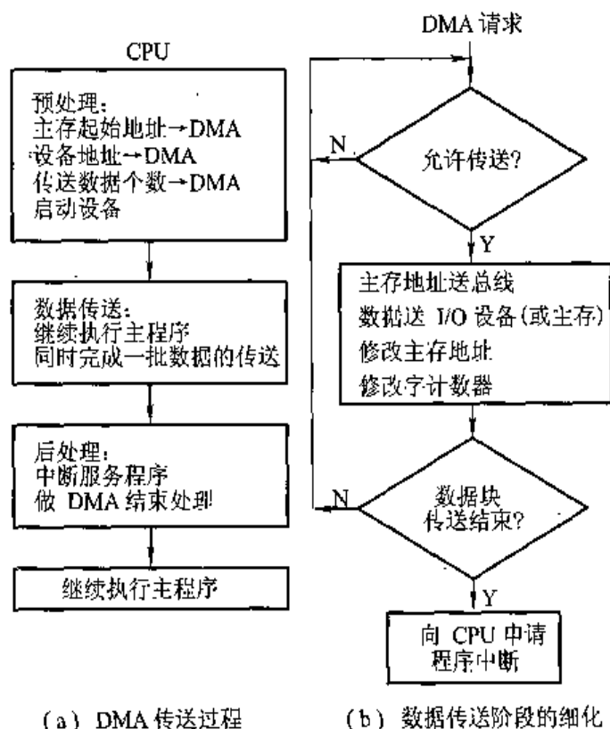
图 5.48 DMA 传送过程示意图
