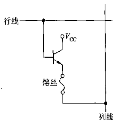
图 4.28 双极型镍铬熔丝式单元电路
