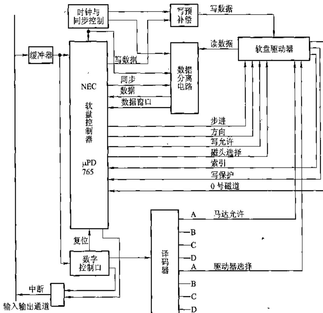
图 4.76 软盘控制器逻辑框图
