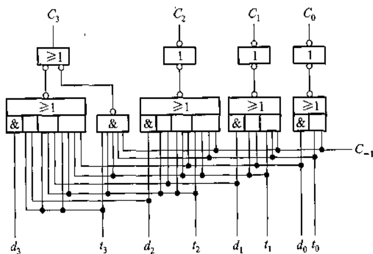
图 6.21 四位一组并行进位链
