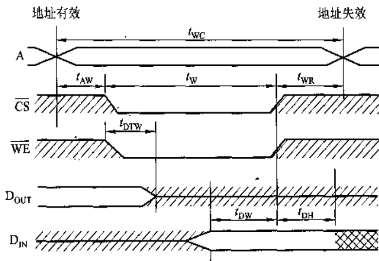
图 4.16 2114 RAM 的写周期时序
