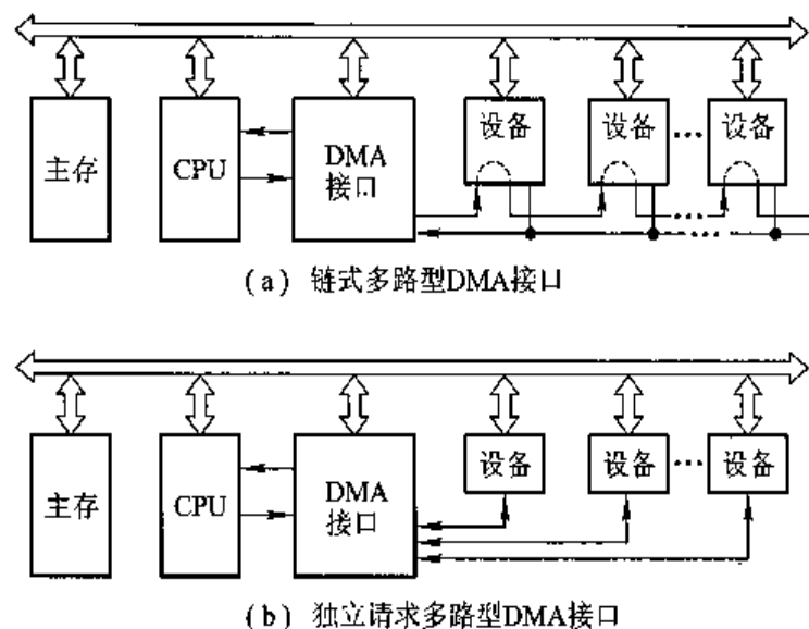
图 5.51 多路型 DMA 接口的逻辑框图
