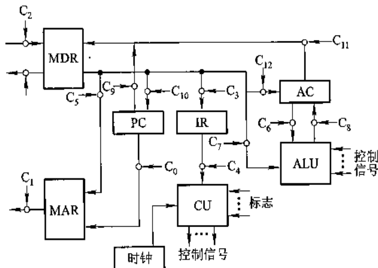
图 9.3 未采用 CPU 内部总线方式的数据通路和控制信号
