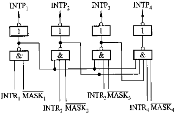
图 8.33 具有屏蔽功能的排队器
