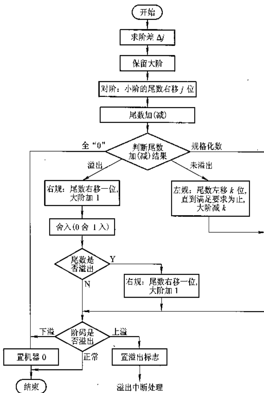
图 6.15 浮点补码加减运算流程
