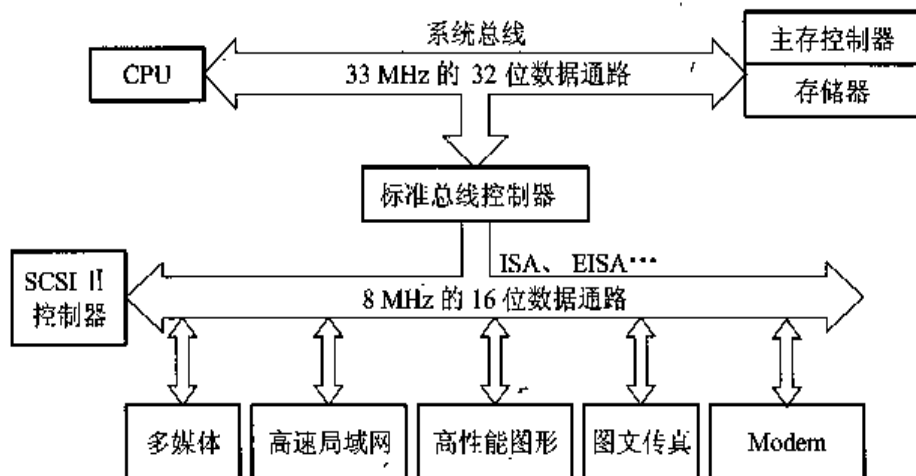
图 3.11 传统微型计算机的总线结构
