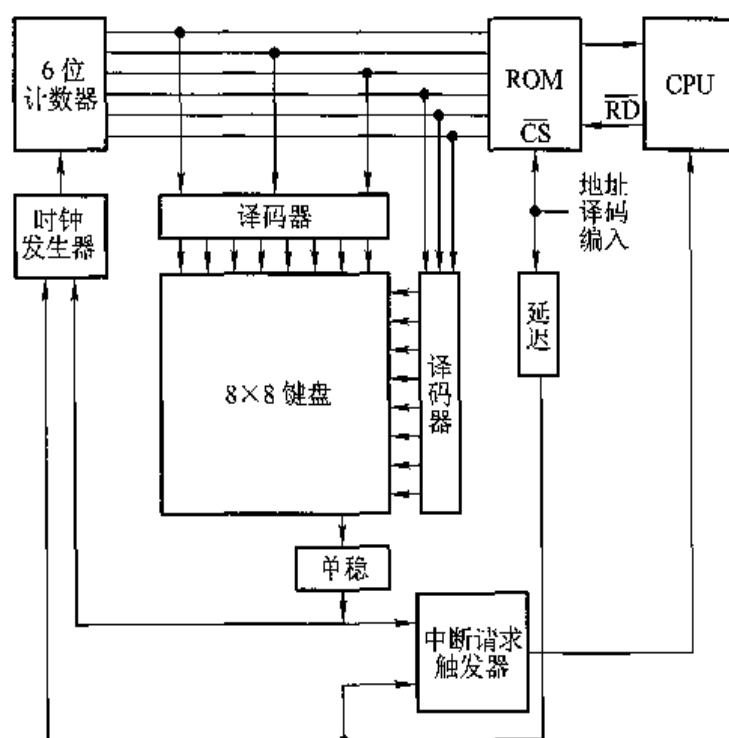
图 5.15 带只读存储器的编码键盘原理图
