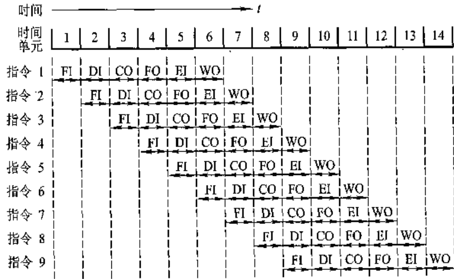
图 8.15 指令六级流水时序
