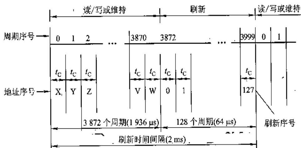
图 4.24 集中刷新时间分配示意图
