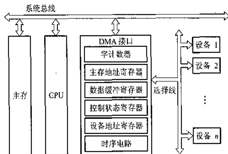
图 5.50 选择型 DMA 接口的逻辑框图
