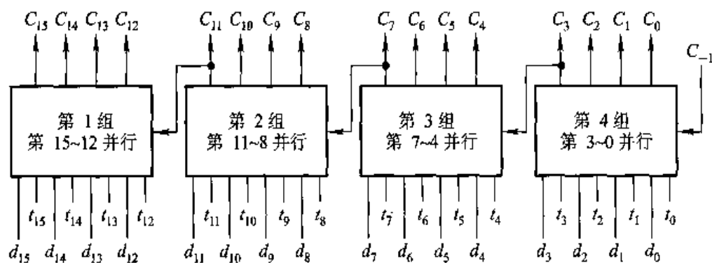
图 6.22 单重分组跳跃进位链框图
