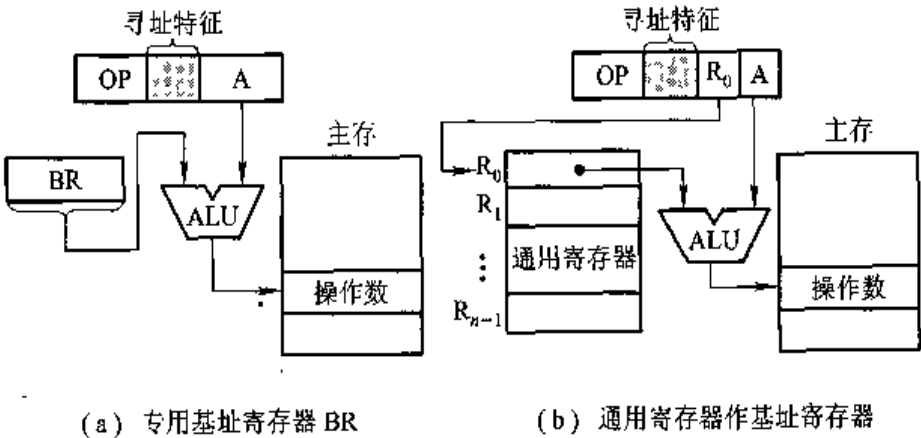
图 7.15 基址寻址示意图
