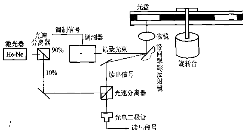
图 4.80 写一次型光盘光学系统的示意图
