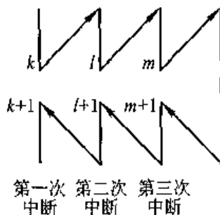
图 8.31 多重中断示意图
