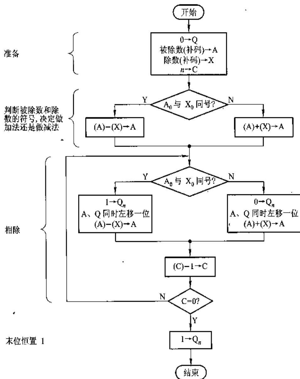
图 6.13 补码加减交替法控制流程
