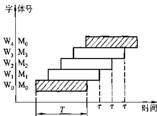
图 4.45 四体低位交叉编址存储器流水线工作方式示意图
