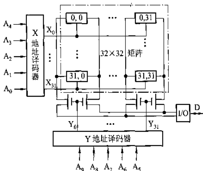
图 4.10 1\text{K} \times 1 位重合法结构示意图
