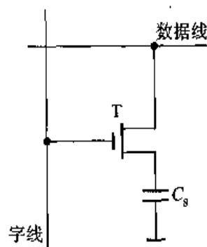
图 4.18 单管 MOS 动态 RAM 基本单元电路
