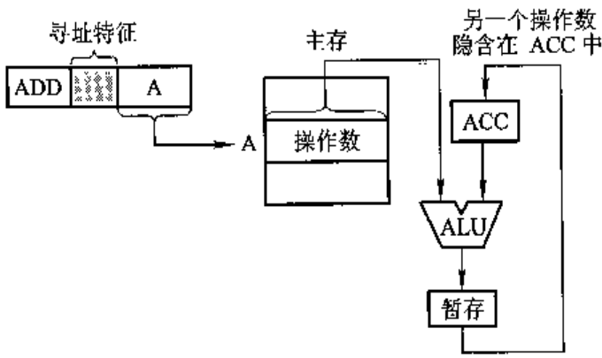
图 7.10 隐含寻址示意图
