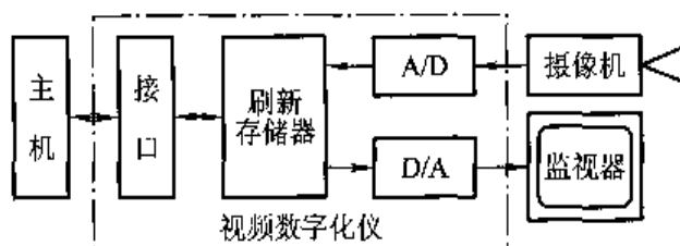
图 5.21 简单的图像显示器原理框图
