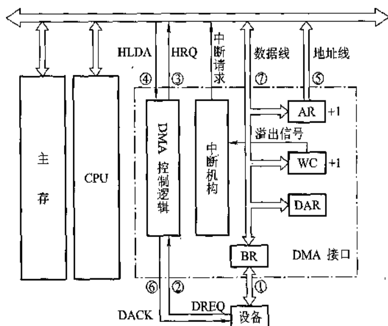
图 5.47 简单的 DMA 接口组成原理图
