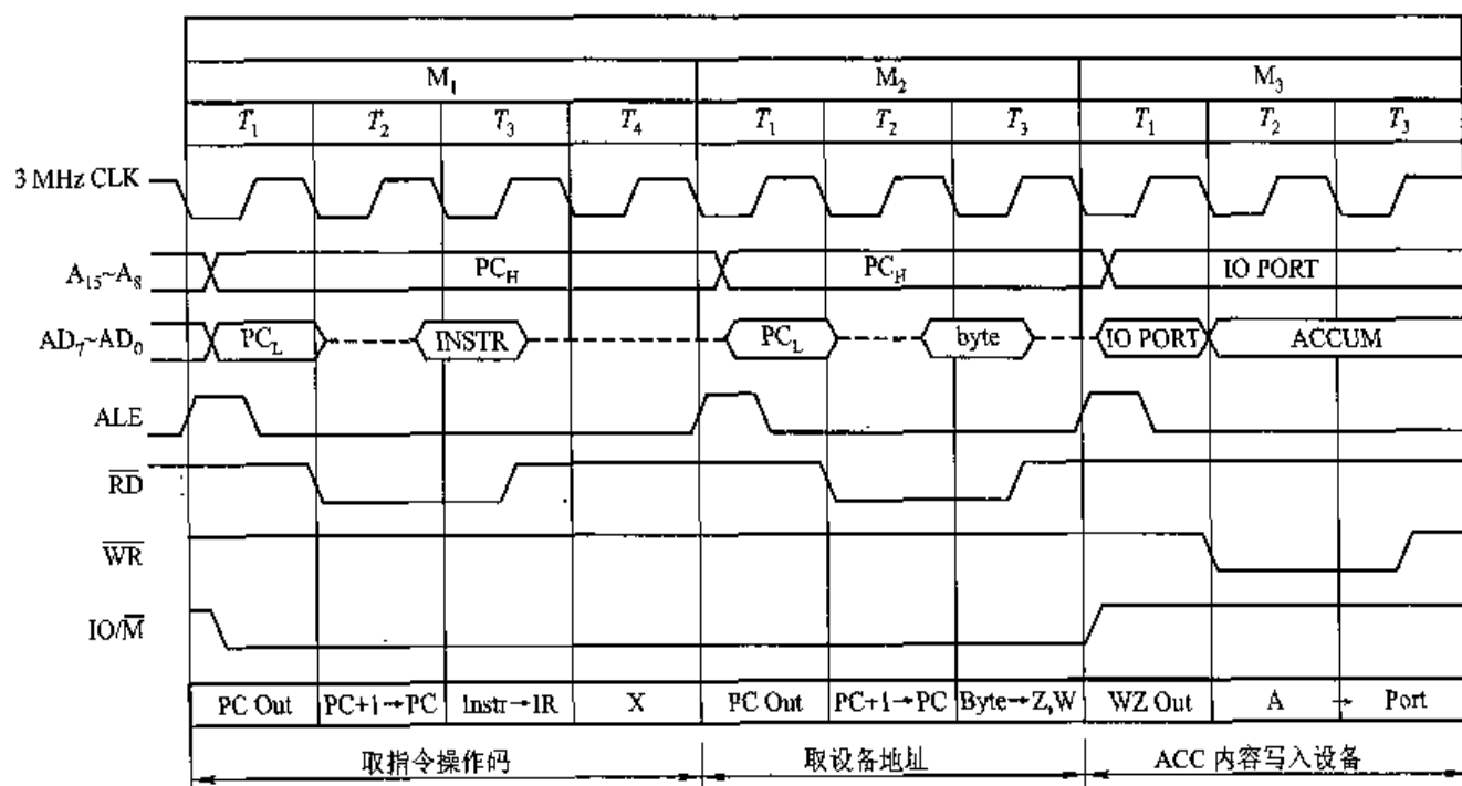
图 9.14 8085 输出指令时序图
