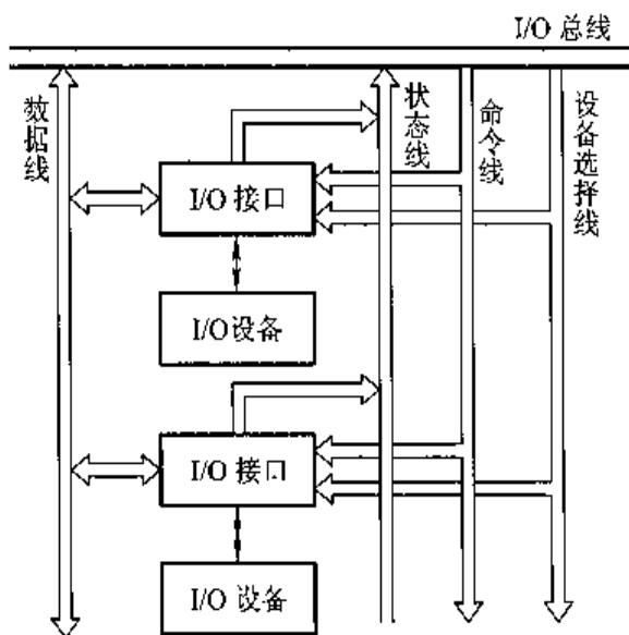
图 5.28 I/O 总线和接口部件
