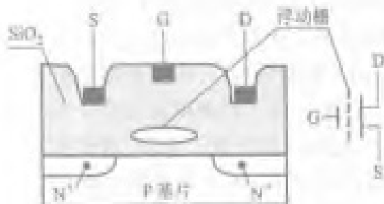
图 4.30 N 型沟道浮动栅 MOS 电路
