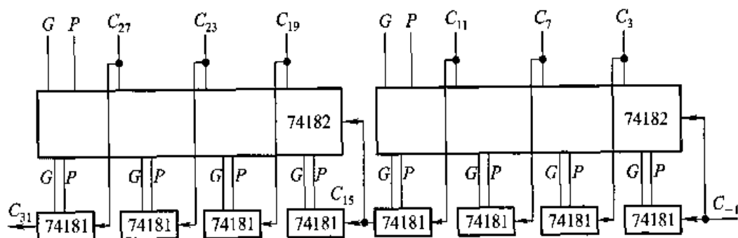
图 6.27 由 74181 和 74182 组成双重分组跳跃进位链
