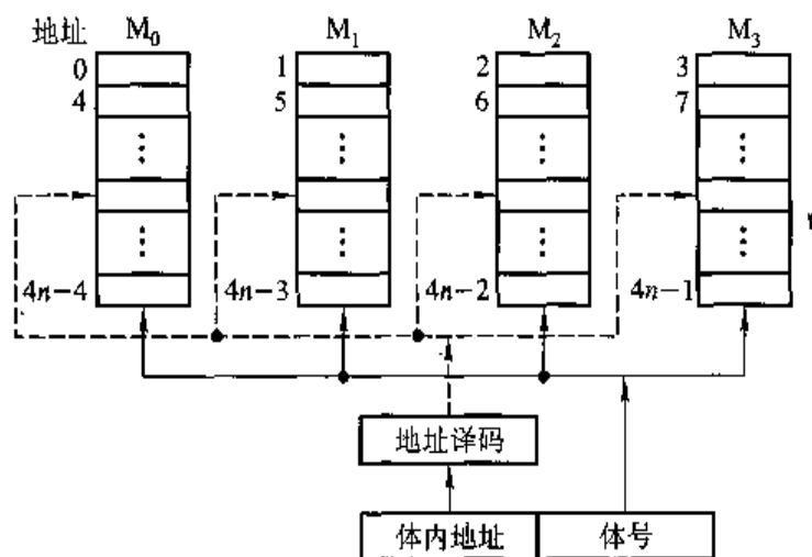
图 4.43 低位交叉编址的多体存储器
