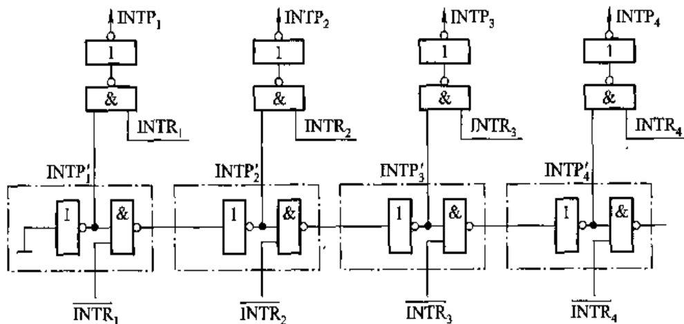
图 5.38 链式排队器
