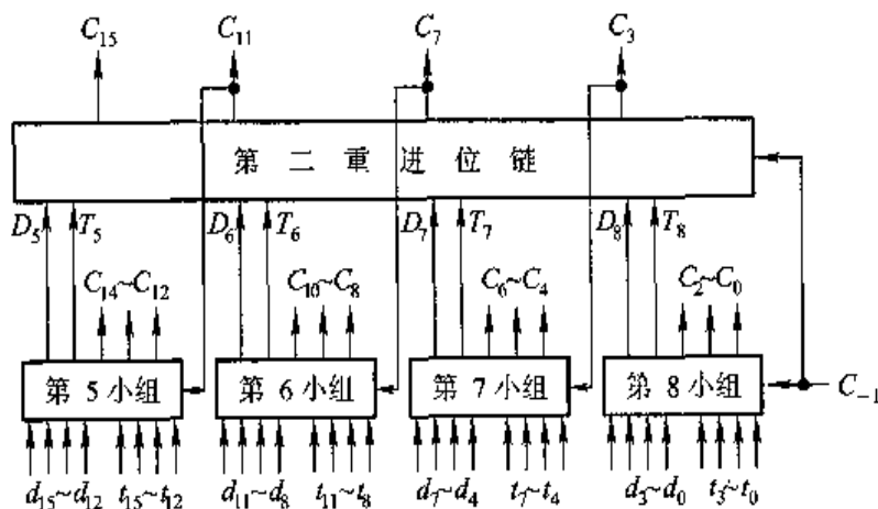
图 6.26 16 位并行加法器的双重分组跳跃进位链框图
