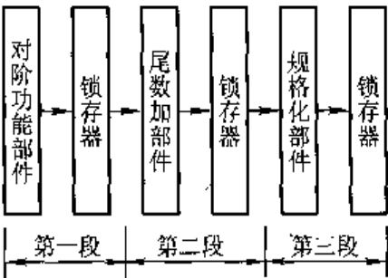
图 8.22 浮点加运算操作流水线
