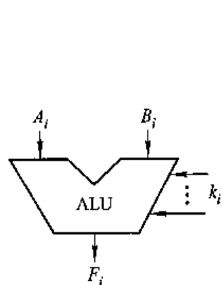
图 6.16 ALU 框图
