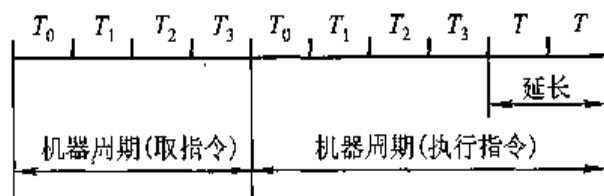
图 9.10 延长机器周期示意
