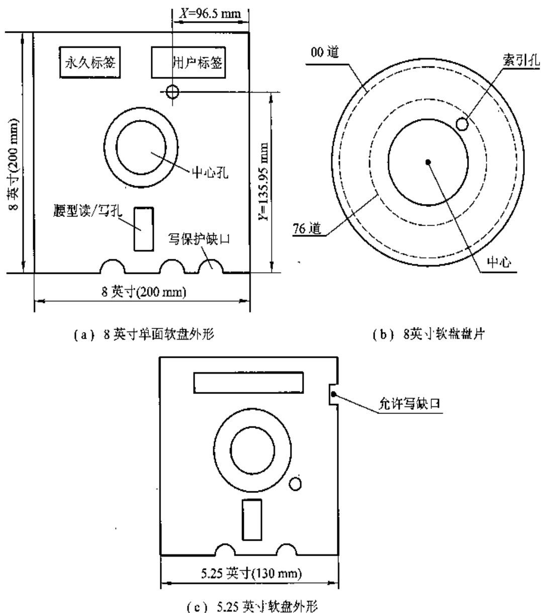
图 4.74 软磁盘盘片及外形
