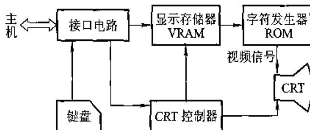
图 5.18 字符显示器原理框图
