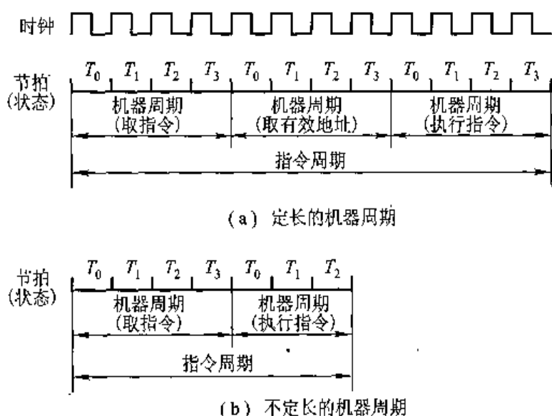
图 9.9 指令周期、机器周期、节拍和时钟周期的关系
