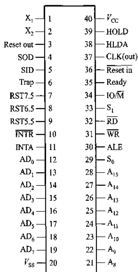
图 9.13 Intel 8085 外部引脚图
