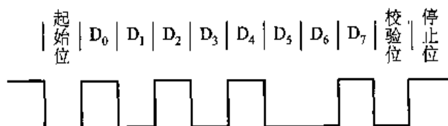
图 3.20 数据 95H 的传送波形
