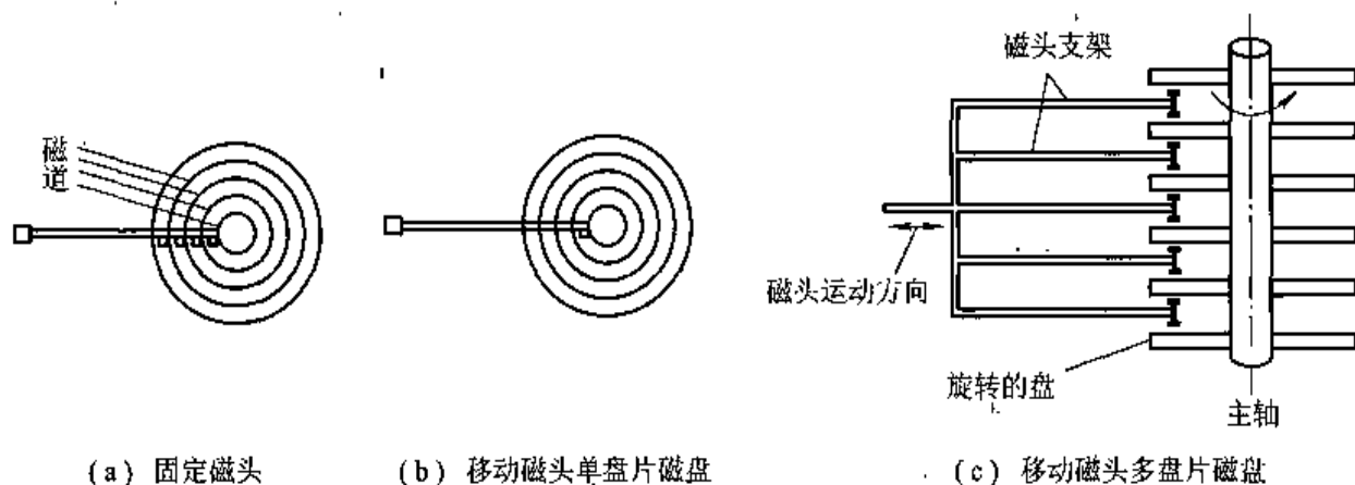
图 4.65 固定头和移动头磁盘
