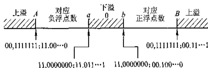
图 6.14 补码在数轴上的表示
