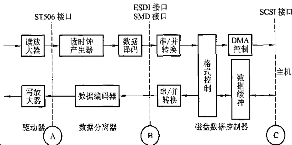
图 4.68 磁盘控制器接口的示意图
