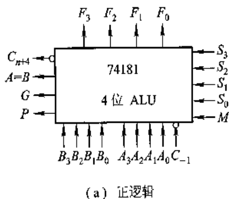
图 6.17 74181 外特性示意图
