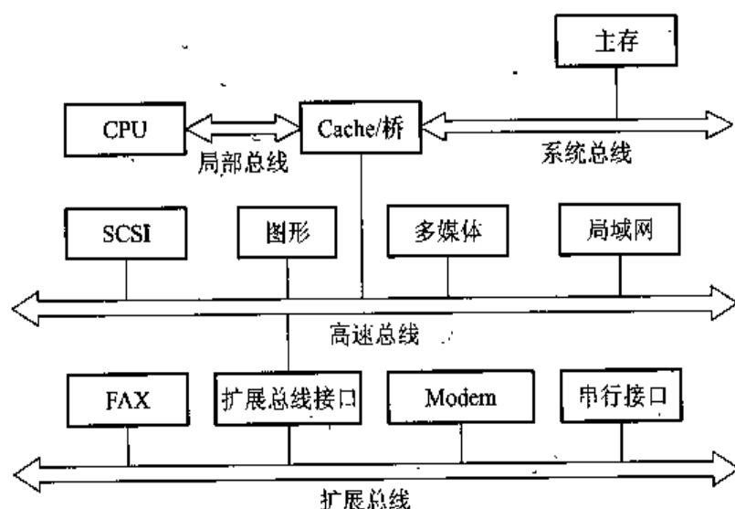
图 3.10 四总线结构
