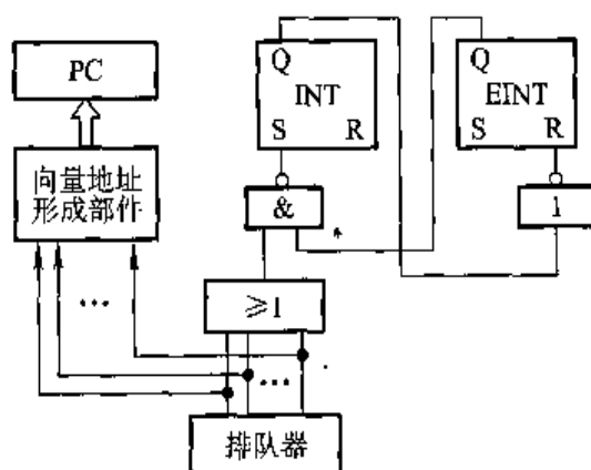
图 8.30 硬件关中断示意图
