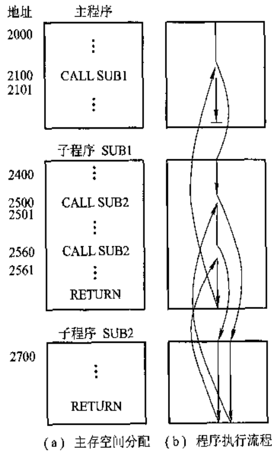
图 7.5 调用和返回指令示意图
