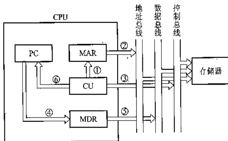
图 8.12 中断周期数据流
