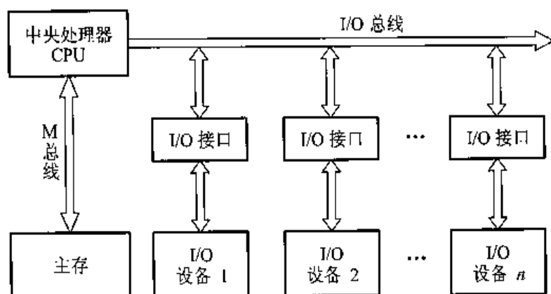
图 3.1 面向 CPU 的双总线结构框图
