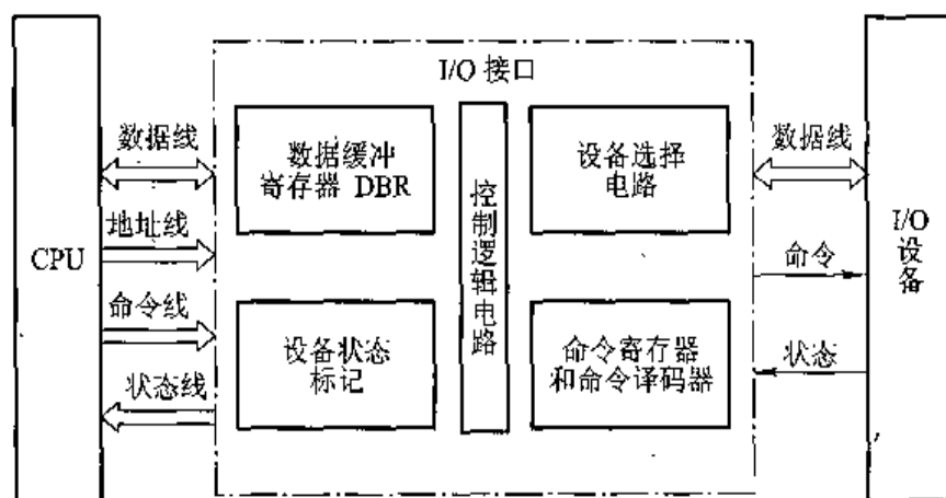
图 5.31 I/O 接口的基本组成
