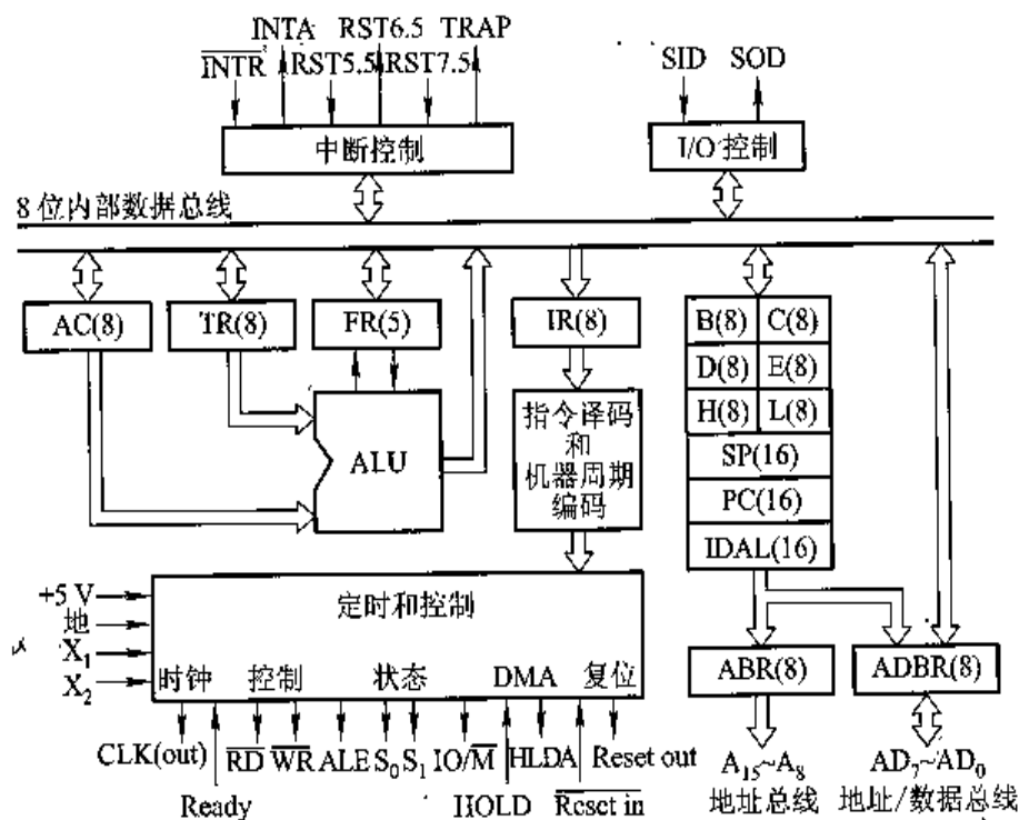
图 9.12 Intel 8085 的组成框图
