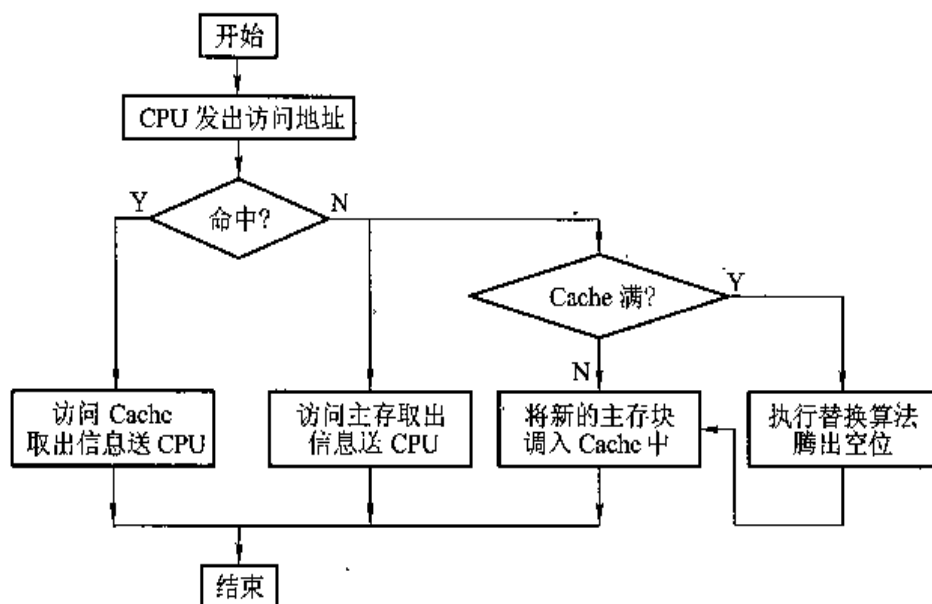
图 4.51 Cache 的读数操作流程
