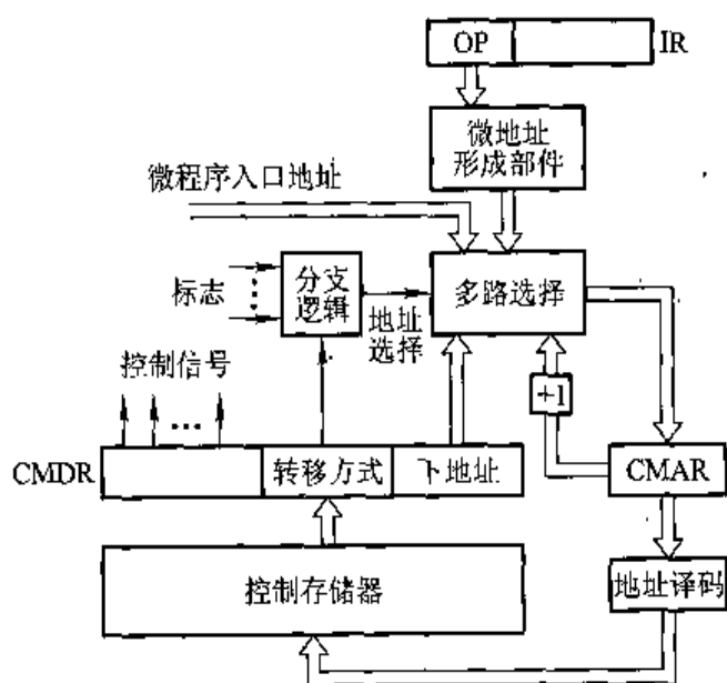
图 10.11 后续微指令地址形成方式的原理图
