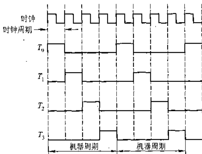
图 9.8 机器周期、时钟周期和节拍的关系
