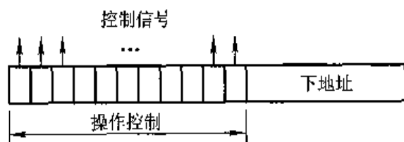
图 10.7 直接编码方式
