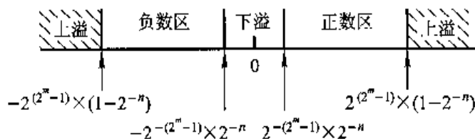
图 6.2 浮点数在数轴上的表示范围
