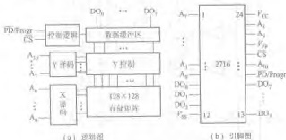
图 4.31 2716 型 EPROM 逻辑图及引脚图
