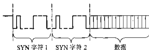
图 3.21 同步串行传送格式
