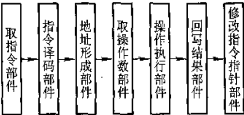
图 8.21 指令流水线结构框图
