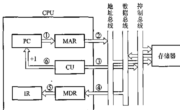
图 8.10 取指周期数据流
