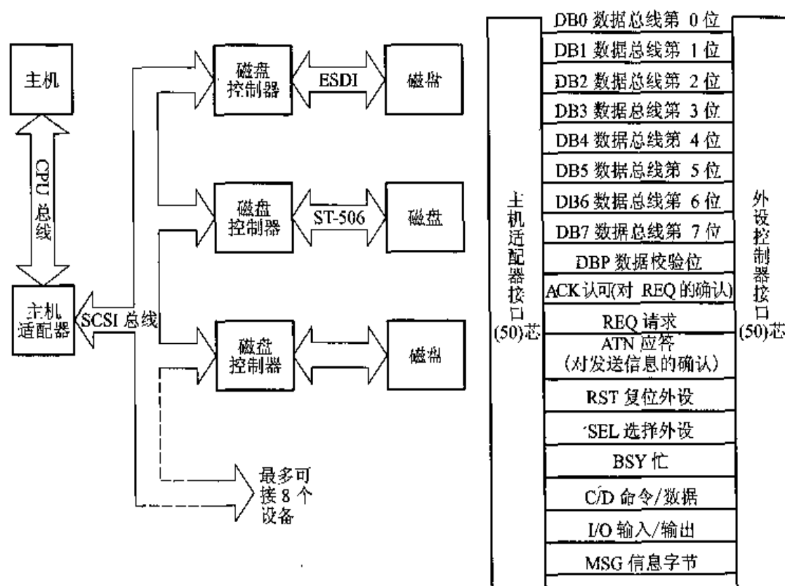
(b) SCSI 接口信号线
