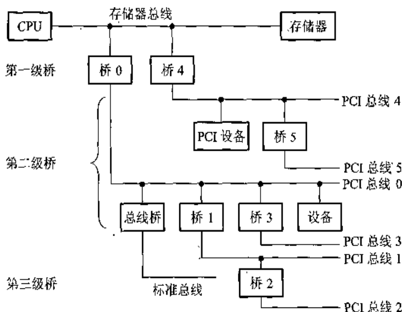
图 3.14 多层 PCI 总线结构
