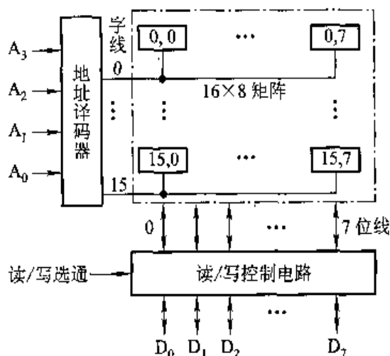
图 4.9 16 \times 1 字节线选法结构示意图
