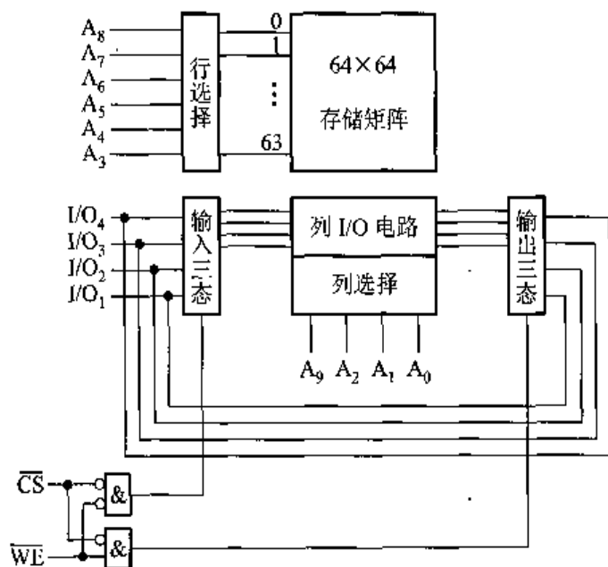
图 4.13 2114 RAM 芯片结构示意图
