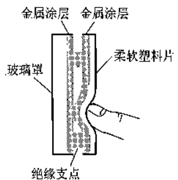
图 5.16 电阻式触摸屏原理
