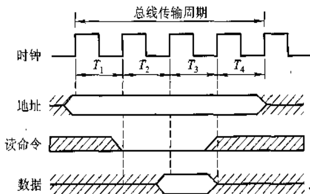
图 3.16 同步式数据输入传输
