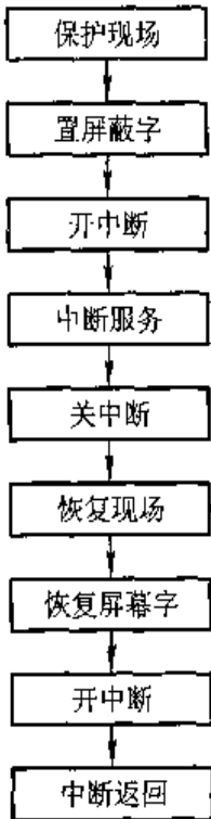
图 8.36 采用屏蔽技术的中断服务程序
