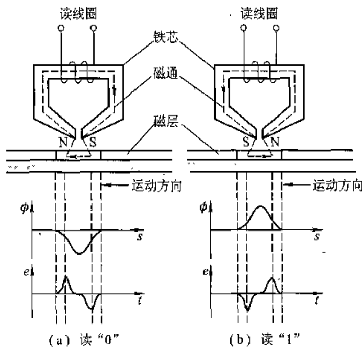
图 4.62 磁表面存储器读出原理
