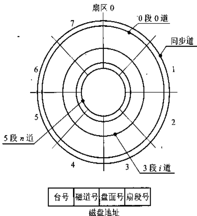
图 4.70 数据在盘片上的分布及磁盘地址定位
