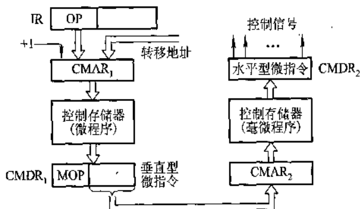
图 10.14 毫微程序控制存储器的基本组成
