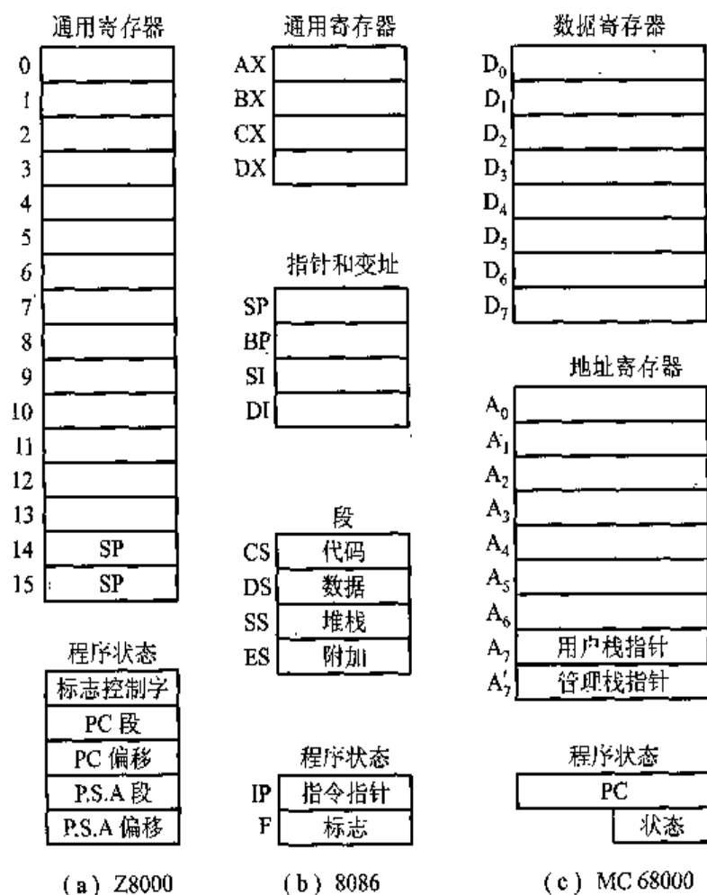
图8.3 三种微处理器的寄存器组织
