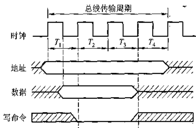
图 3.17 同步式数据输出传输
