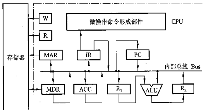
图 10.2 例 10.1 CPU 内部结构框图
