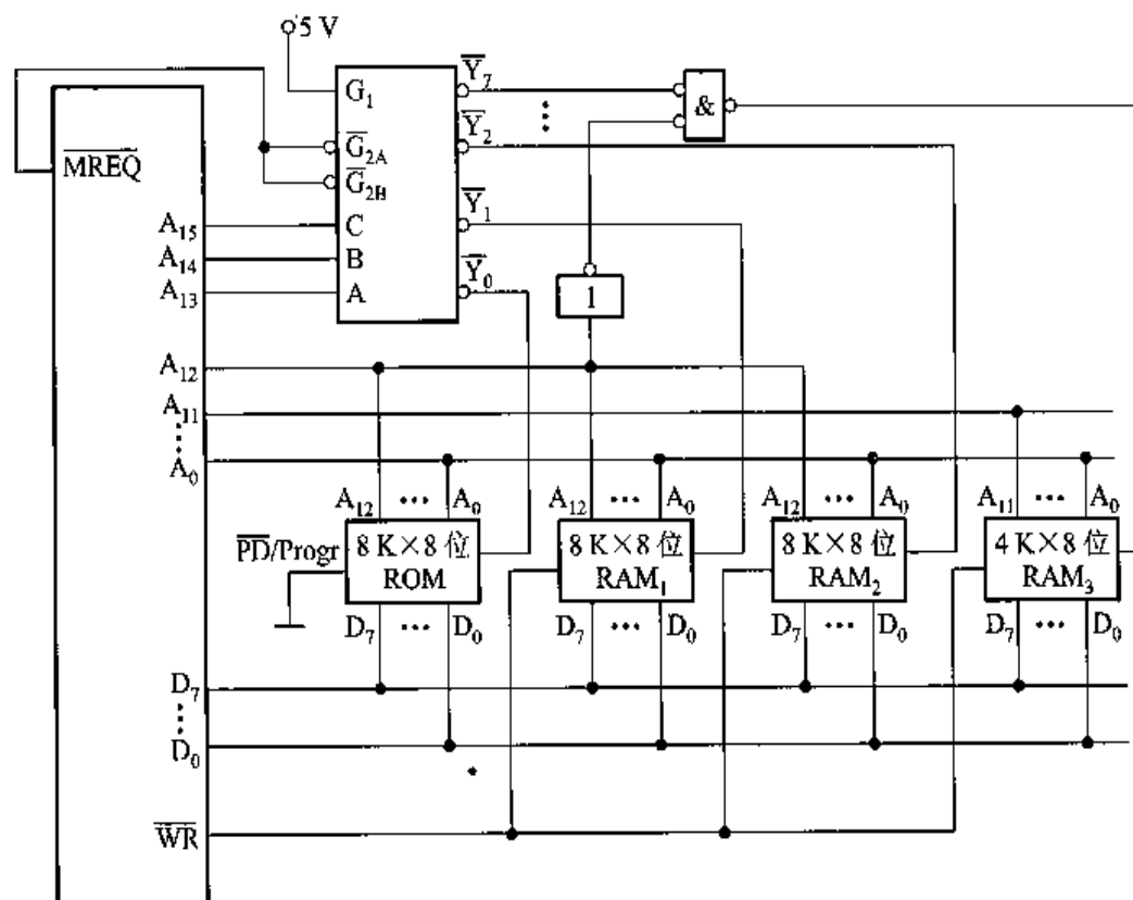
图 4.38 例 4.2 CPU 与存储芯片的连接图
