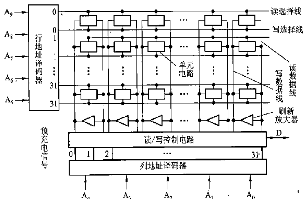
图 4.19 1K x 1 位三管 MOS 动态 RAM 结构示意图
