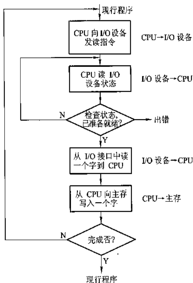
图 5.9 程序查询方式流程
