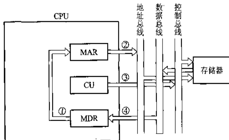
图 8.11 间址周期数据流
