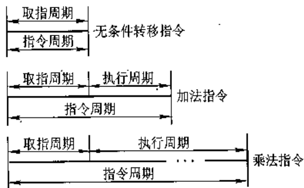
图 8.6 各种指令周期的比较
