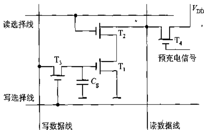
图 4.17 三管 MOS 动态 RAM 基本单元电路
