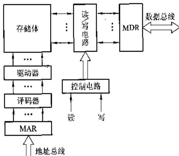
图 4.4 主存的基本组成
