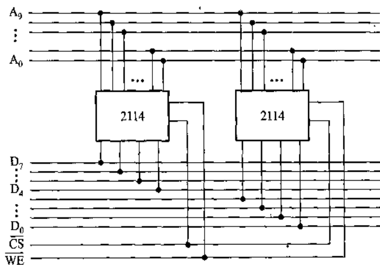
图 4.32 由 2 片 1\text{ K} \times 4 位的芯片组成 1\text{ K} \times 8 位的存储器
