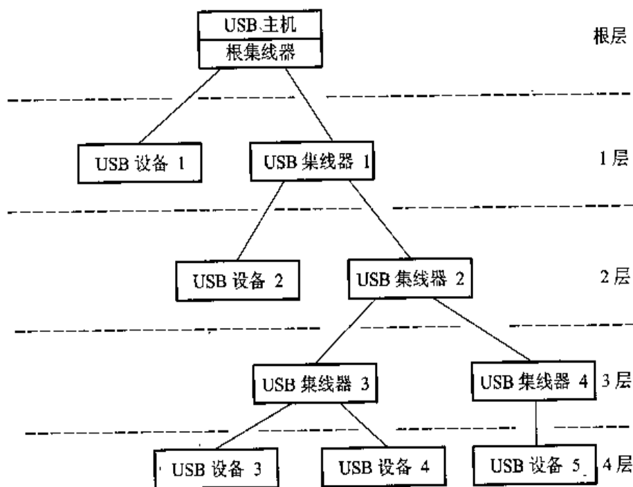
图 3.6 典型的 USB 系统拓扑结构
