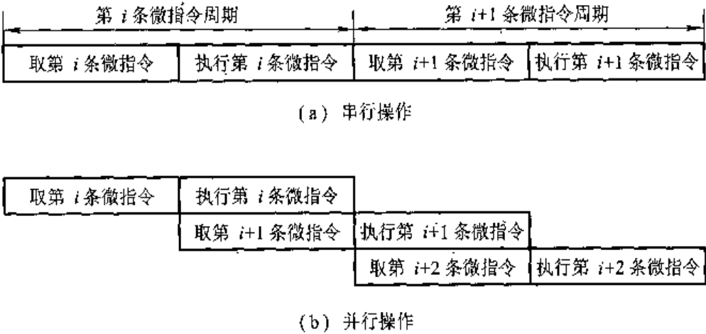
图 10.15 串行微程序和并行微程序控制方式
