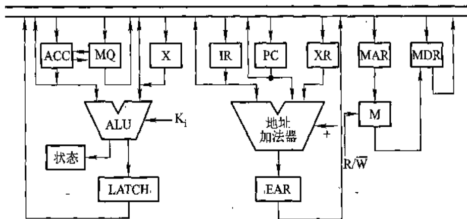
图 9.5 单总线计算机结构
