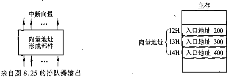
图 8.27 集中在 CPU 内的向量地址形成部件
