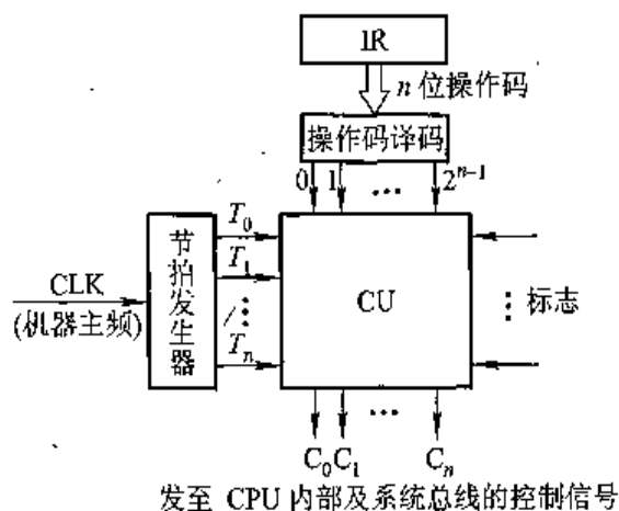
图 10.1 带译码和节拍输入的控制单元框图
