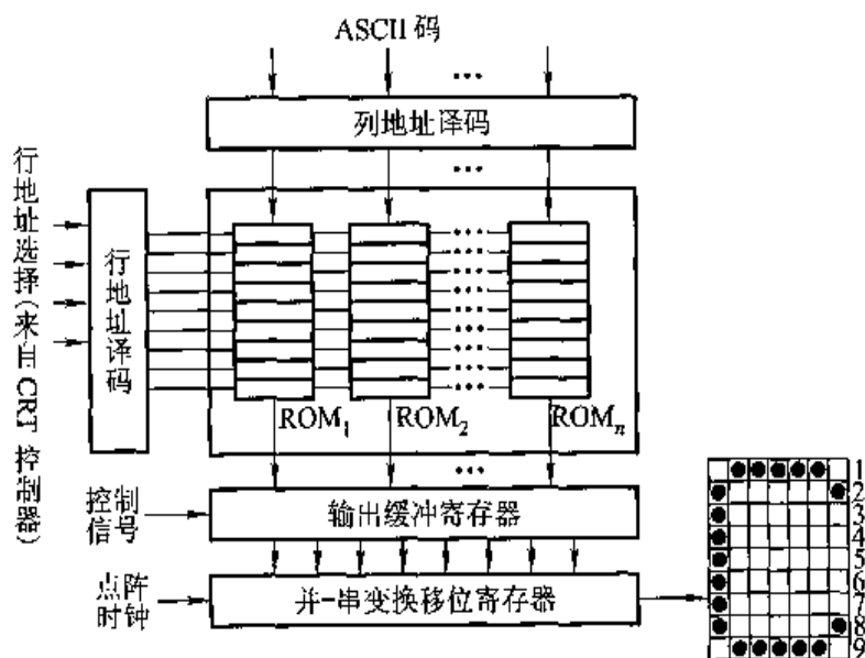
图 5.19 对应 7 \times 9 光点矩阵的字符发生器原理图
