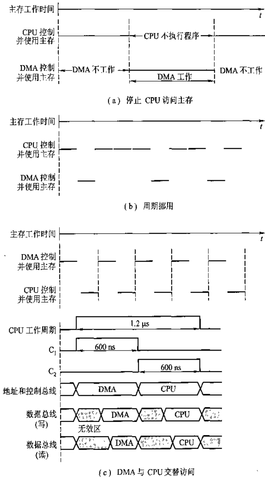
图 5.46 DMA 的三种传送方式
