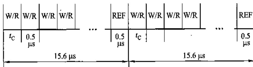
图 4.26 异步刷新时间分配示意图
