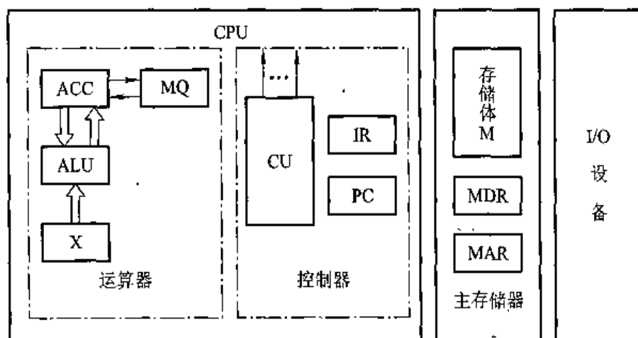
图 1.11 细化的计算机组成框图
