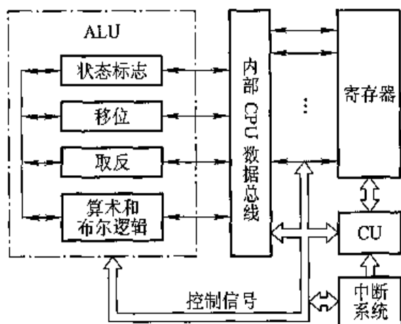
图 8.2 CPU 的内部结构
