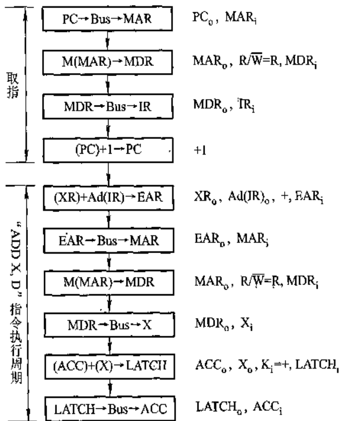
图 9.6 “ADD X,D”指令周期的信息流程及相应的控制信号
