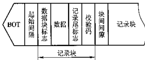
图 4.78 磁带的格式
