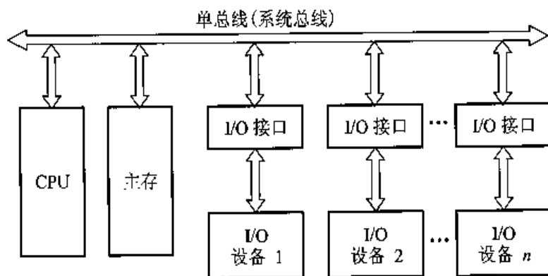
图 3.2 单总线结构框图
