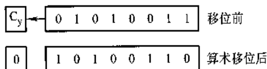
图 6.4 用带进位的移位实现算术左移
