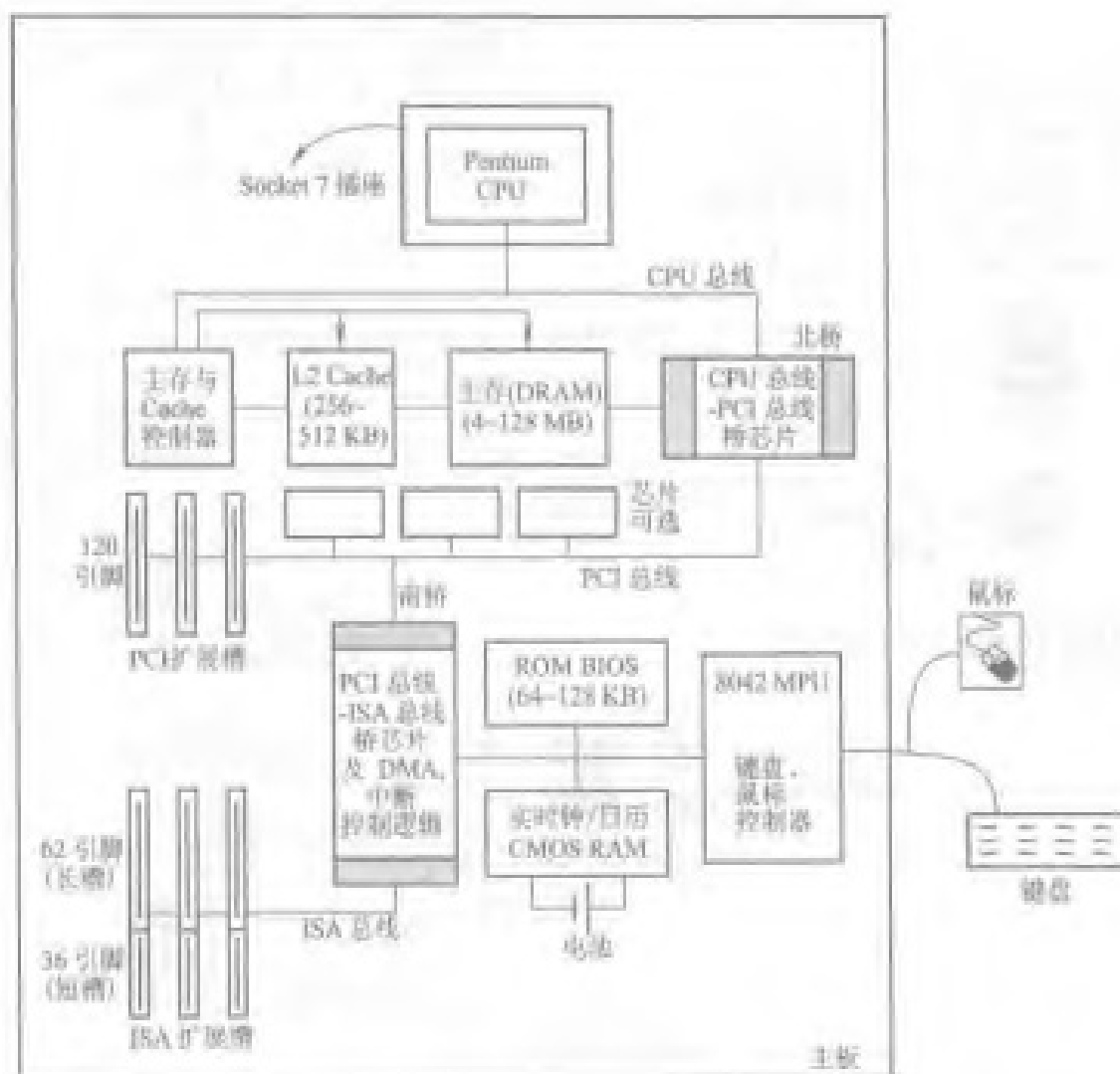
图 10.19 Pentium 主板结构示意图
