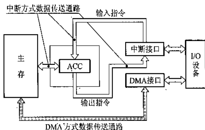
图 5.45 DMA 和程序中断两种方式的数据通路
