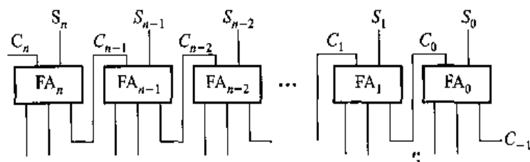
图 6.19 并行加法器示意图
