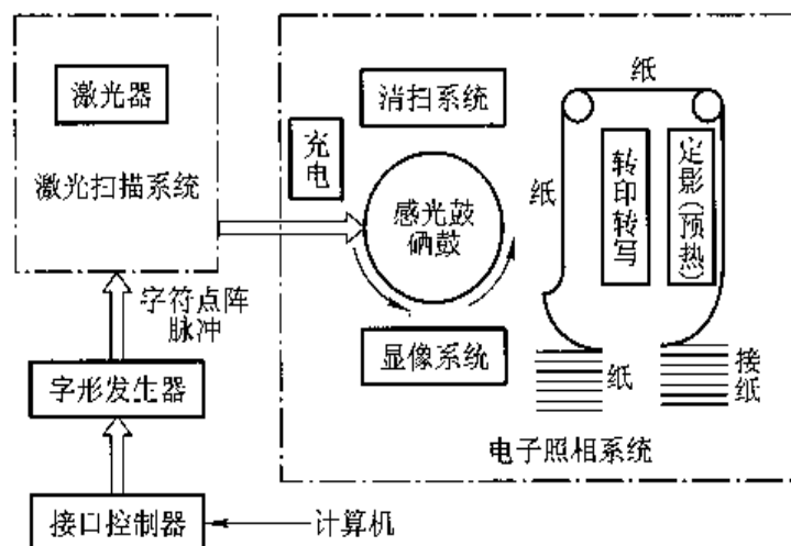
图 5.24 激光打印机原理框图
