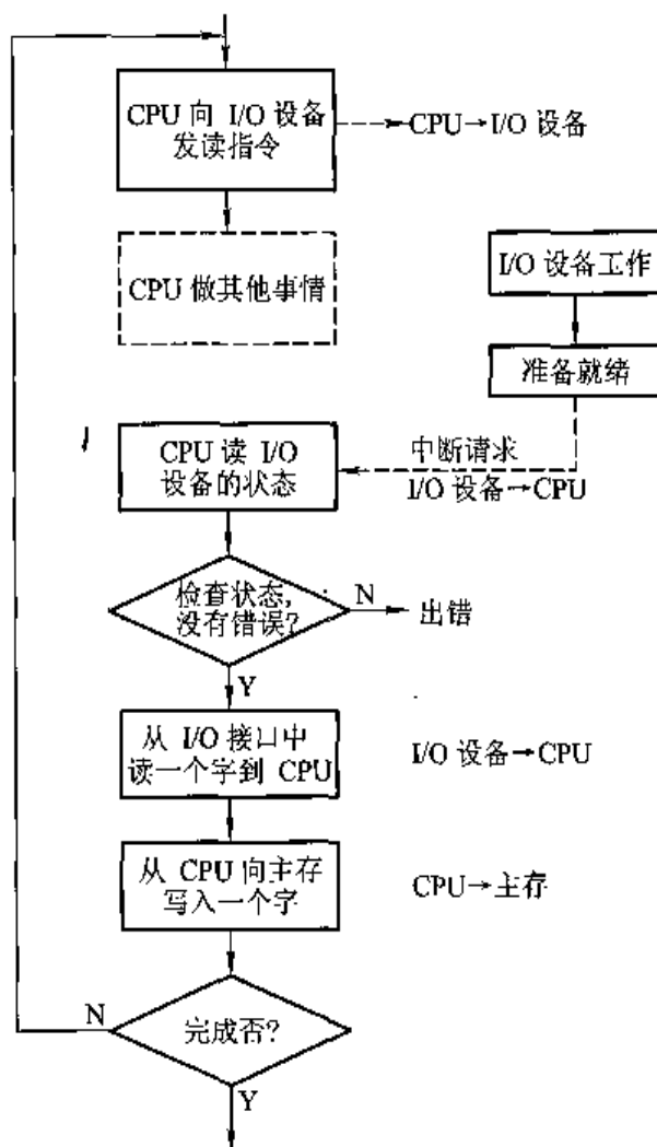
图 5.11 程序中断方式流程
