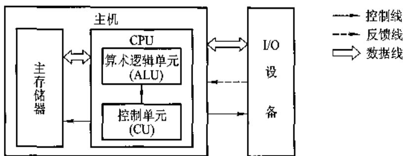
图 1.9 现代计算机的组成框图
